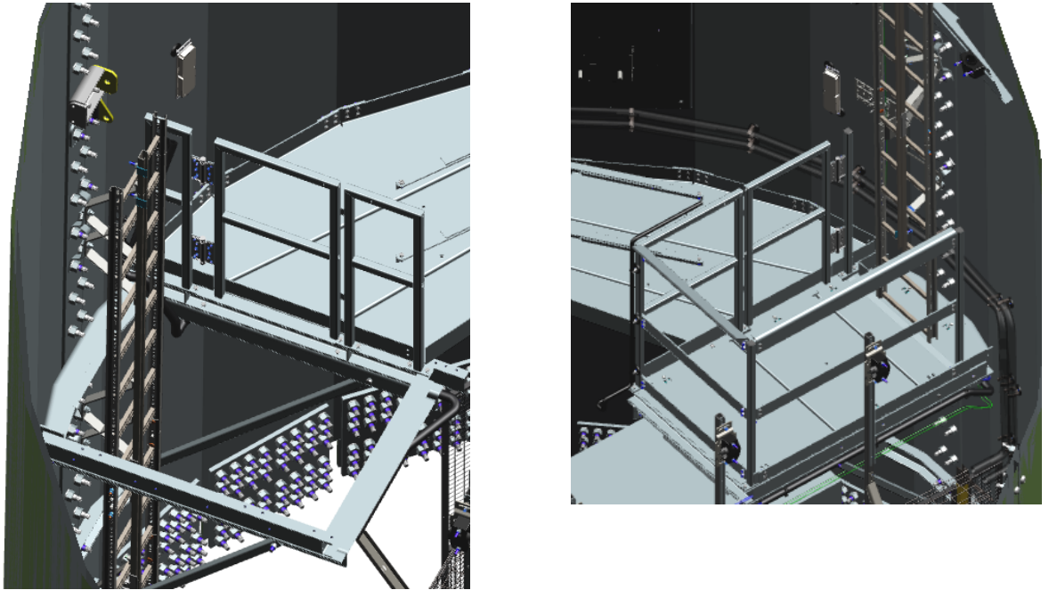
Abb. 12: Zugang zum Mittelspannungsraum (links), Landepodest der Aufstiegshilfe (rechts) (Beispiel)
