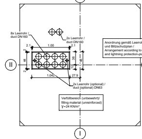
Detail 2 Maßstab / Scale 1:25 Angaben in [mm]
