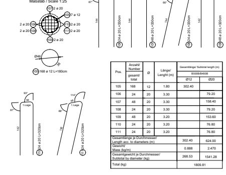
Schnitt / Section B-B Maßstab / Scale 1:25
