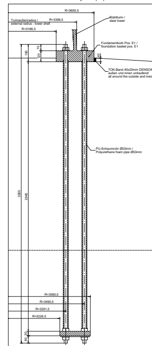
Detail 1 Maßstab / Scale 1:10 Angaben in [mm]
