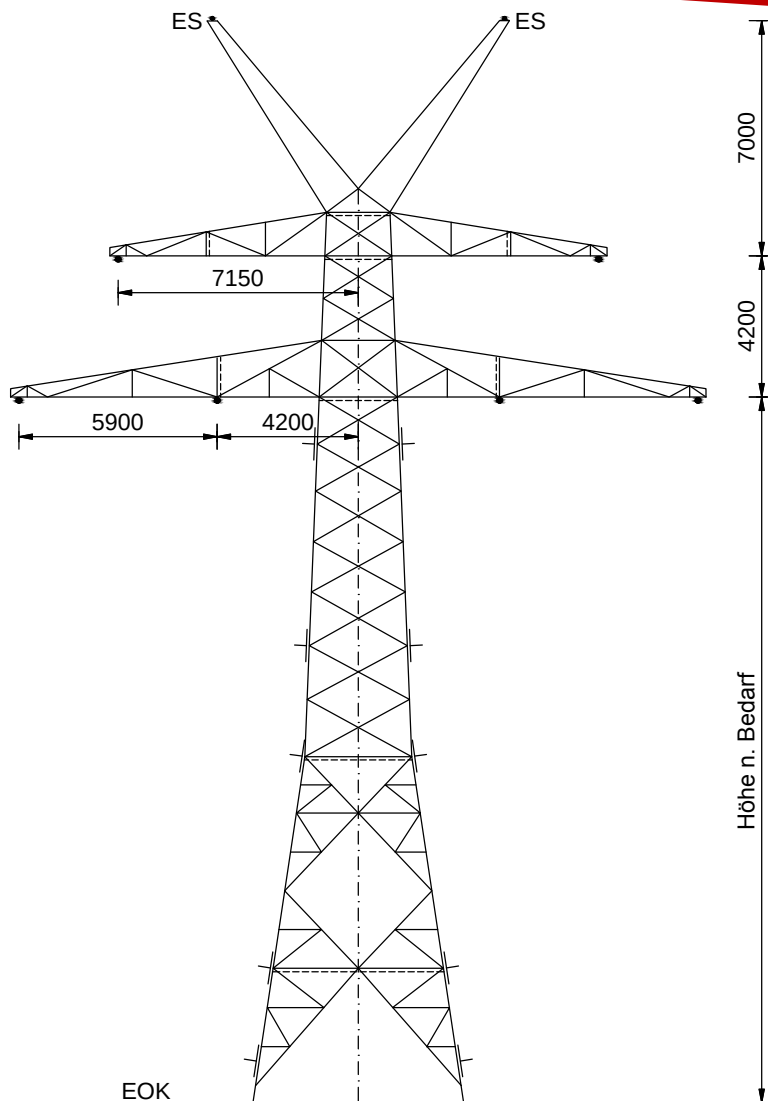
Abspannmast WE100
