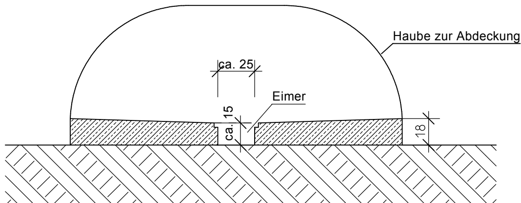
Schnitt
