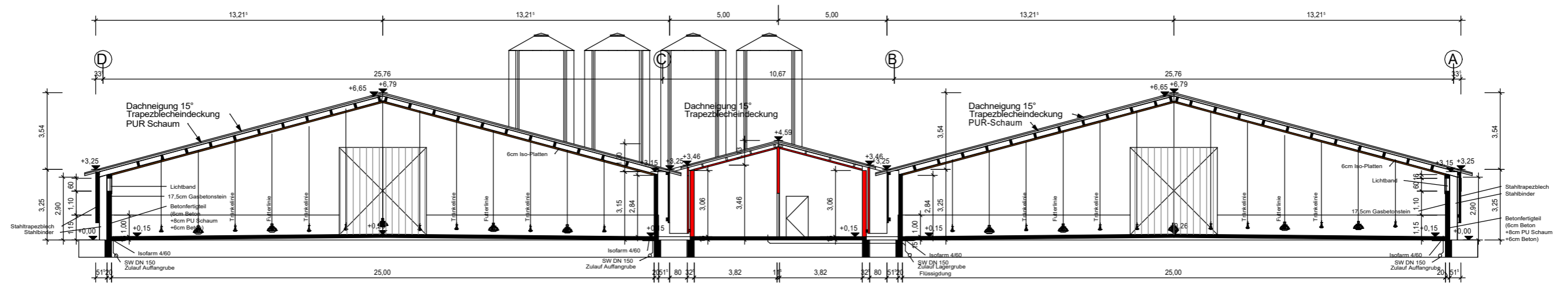
Schnitt A - A
