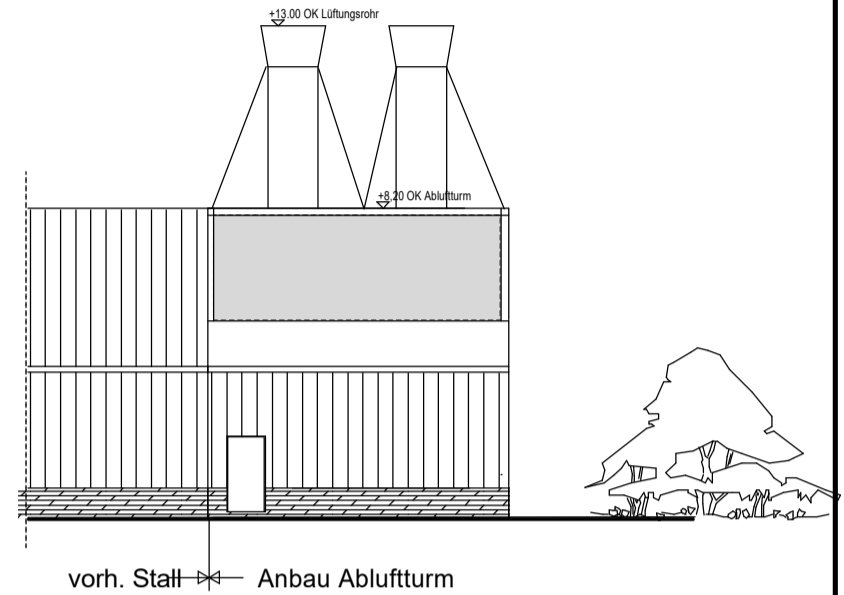
Südansicht Stall 1
