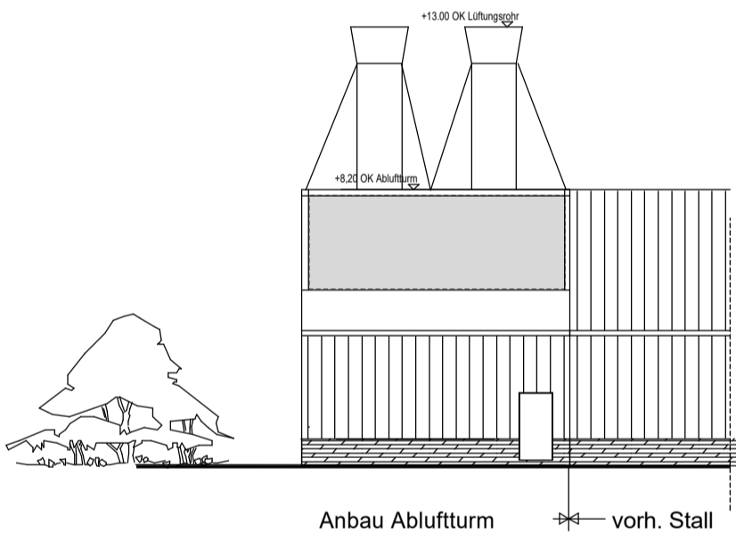
Nordansicht Stall 2
