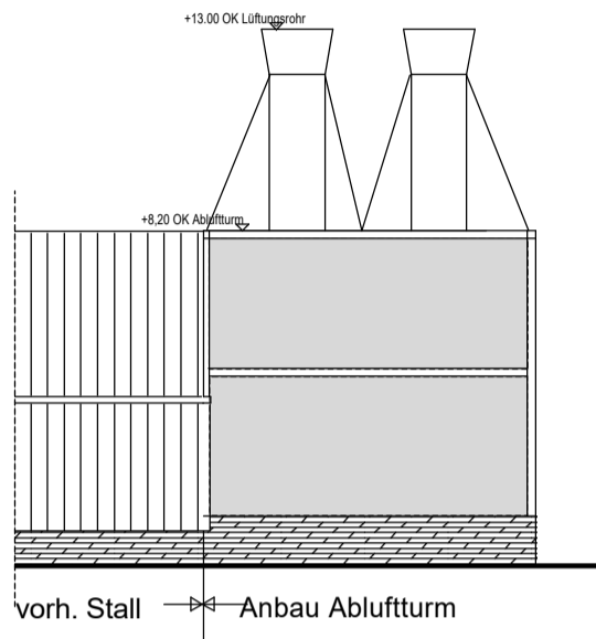
Südansicht Stall 2
