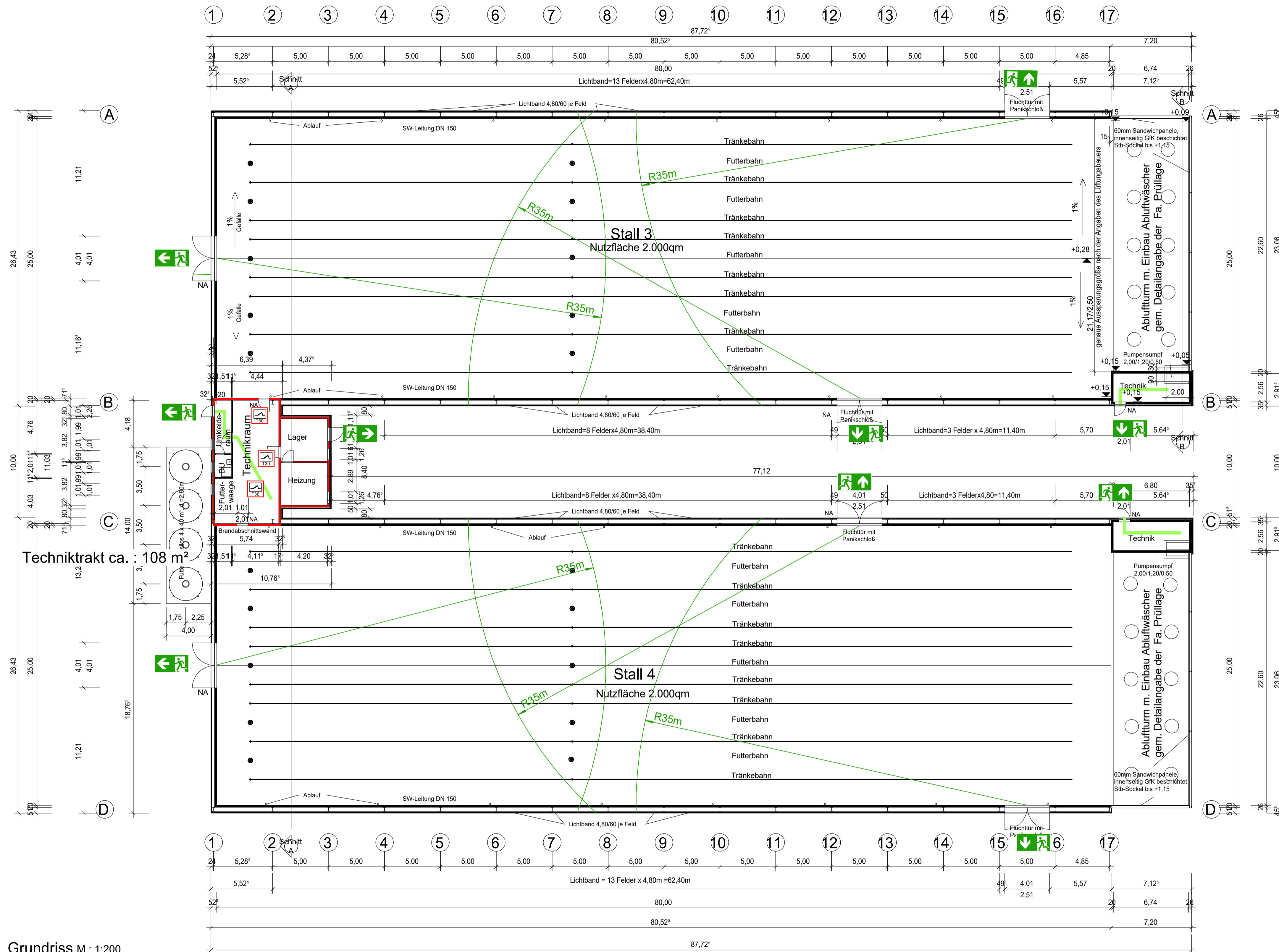
Grundriss, M.: 1:200
