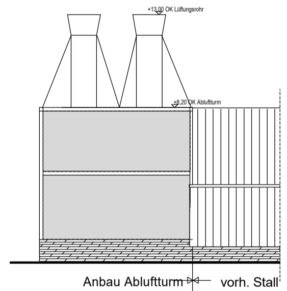
Nordansicht Stall 1
