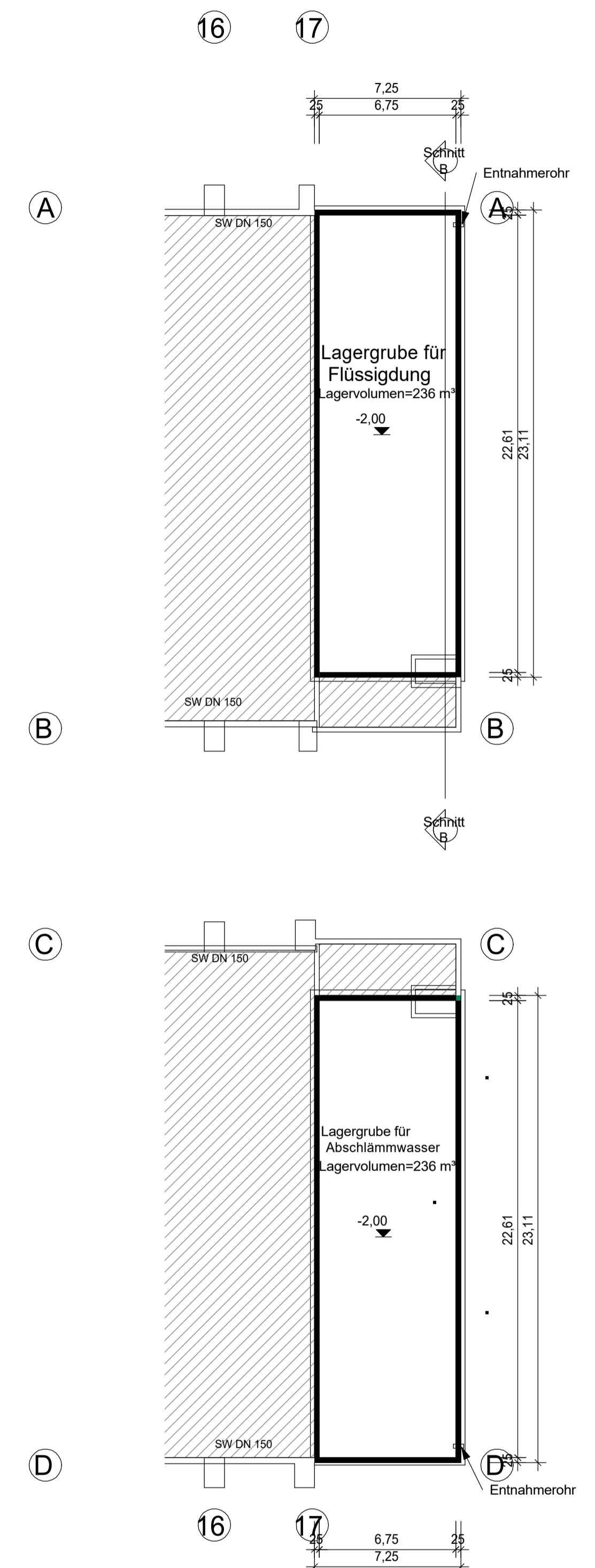
Grundriss Lagergrube ,M.: 1:200
