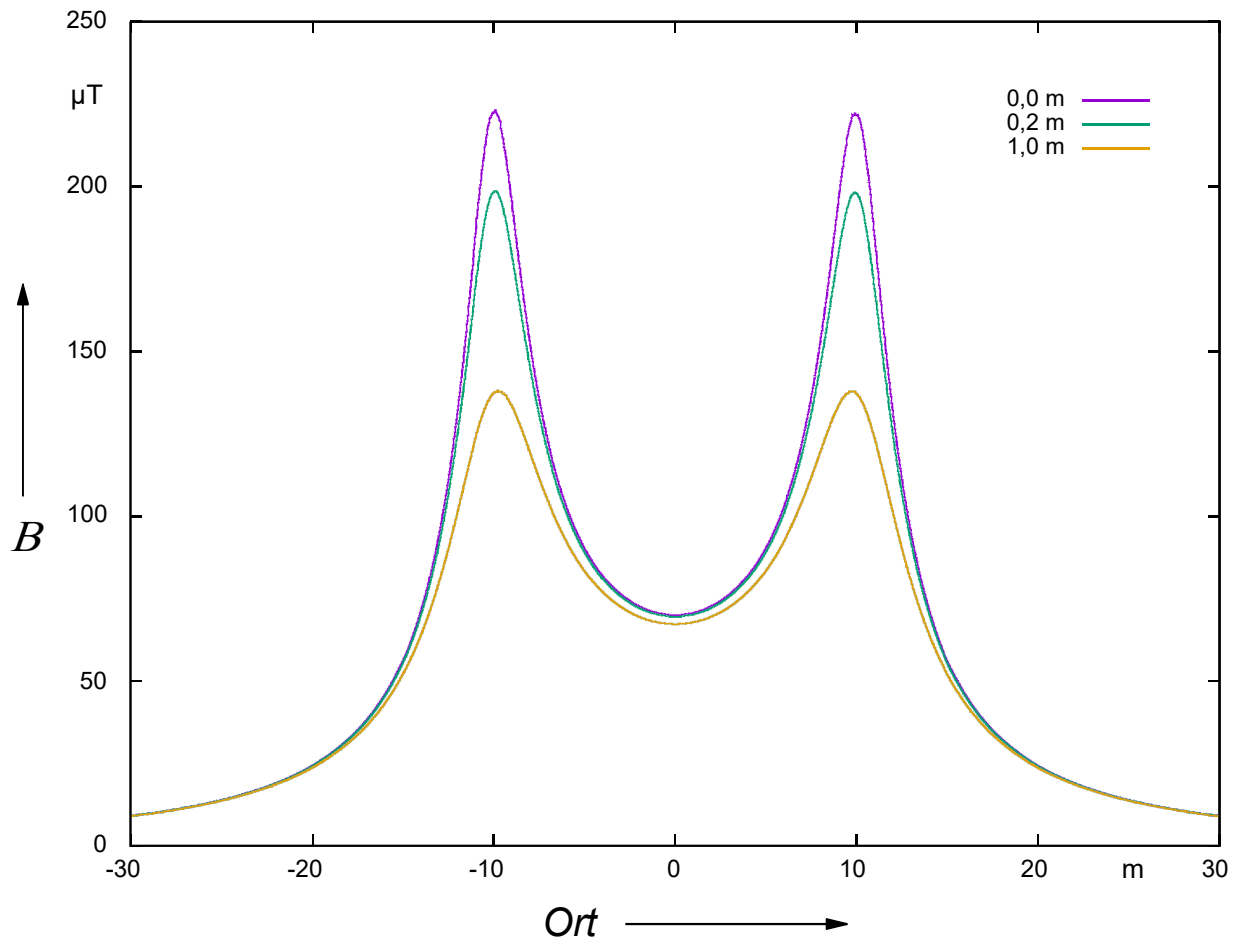
Abb. 23: Magnetische Flussdichten in unterschiedlichen Entfernungen, Polabstand 20,0 m, Überdeckung 1,5 m, Leiterquerschnitt 2500 mm 2 , 1905 A
