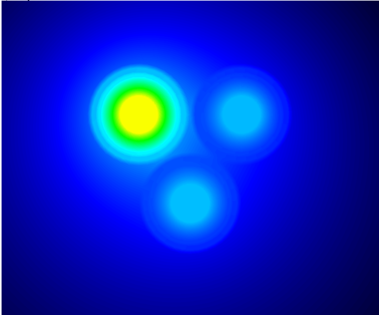
Abb. 11: Temperaturverteilungen in der Kabelanlage bei a) beide Pole stromführend, b) ein Pol stromlos und c) ein Pol halber Strom
