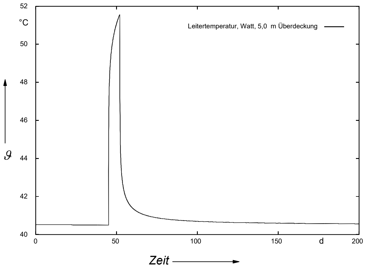
Abb. 7: Leitertemperaturverlauf, trockenfallendes Watt, Überdeckung 5,0 m, Leiterquerschnitt 2500 mm 2
