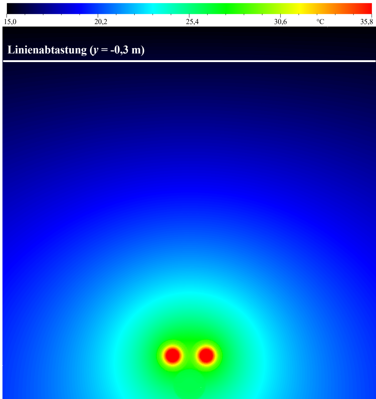
Abb. 26: Temperaturverteilung im stationären Vorzustand, FEM-Berechnung
