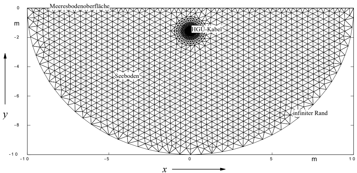
Abb. 3: Finite-Elemente-Modell (Gesamtansicht)
