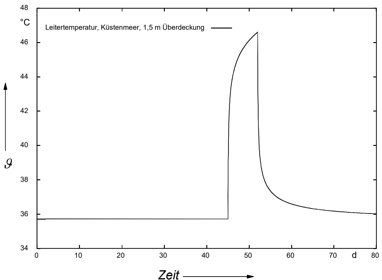
Abb. 12: Temperaturverlauf im Leiter, Küstenmeer, ständige Überflutung, Überdeckung 1,5 m Leiterquerschnitt 2500 \text{ mm}^2
