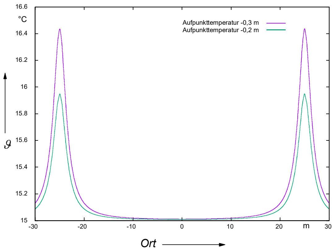
Abb. 10: Linienabtastungen durch die Aufpunkte in 0,2 m und 0,3 m Tiefe, oben ein System, unten beide Systeme in Betrieb, Überdeckung 1,5 m, I = 1467 A
