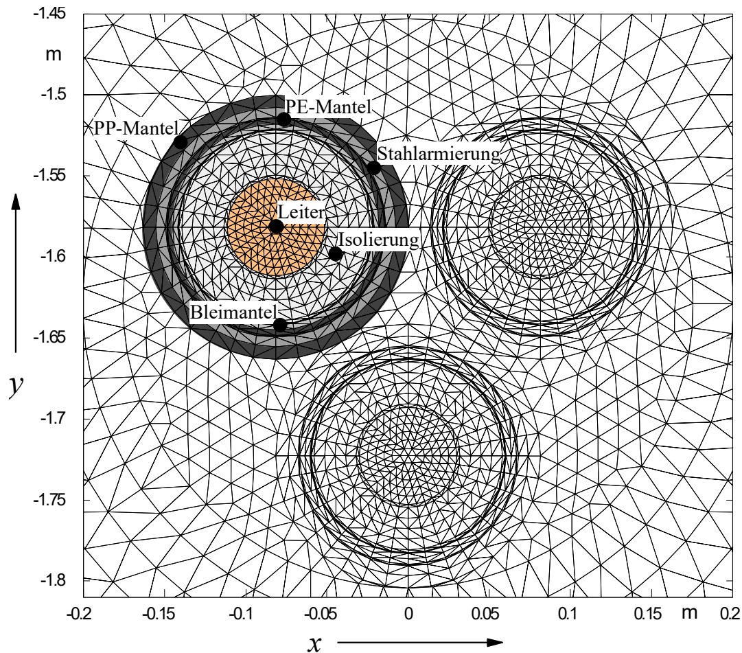
Abb. 4: Finite-Element-Modell, Ausschnittvergrößerung im Bereich des Kabelbündels, Leiterquerschnitt 2500 mm 2
