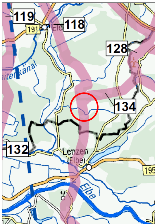
Abbildung 1: Ausschnitt Trassenkorridornetz SuedOstLink+ // Betroffenheit Windenergieanlagen
