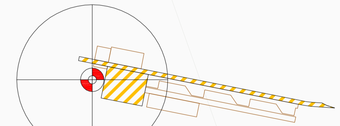
Windenergieanlage (WEA) mit Nr. Typ: Nordex N-163/6.X, 6,8 MW, Rotordurchmesser 163,00 m, Rotorradius 81,50 m, Nabenhöhe 164,00 m, Gesamthöhe 245,50 m mit Zuwegung, Stell- und Montageflächen
