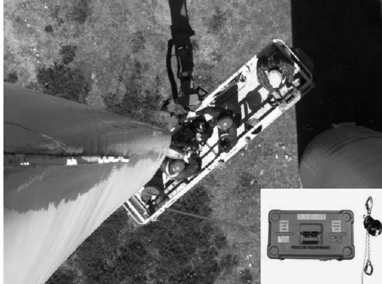
Abbildung 10-1: Beispiel für einen Notabstieg an einem Mannkorb
