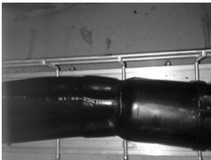
Abbildung 7-1: Risse im Schrumpfschlauch des Mittelspannungskabels.
