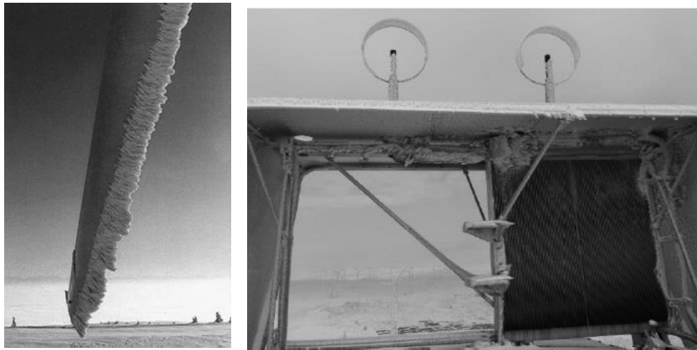
Abbildung 7-2: Ansammlung von Eis auf dem Rotorblatt und Cooler Top®
