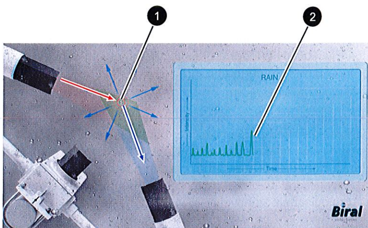
Abb. 2: Messbeispiel Regen
