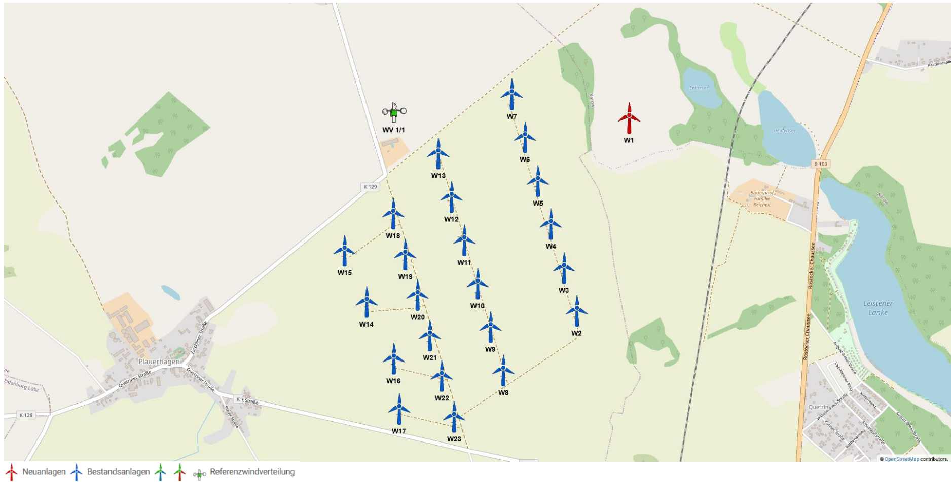
Abbildung 2.1: Zu untersuchende Windparkkonfiguration; Kartenmaterial: [19.1, 19.2]
