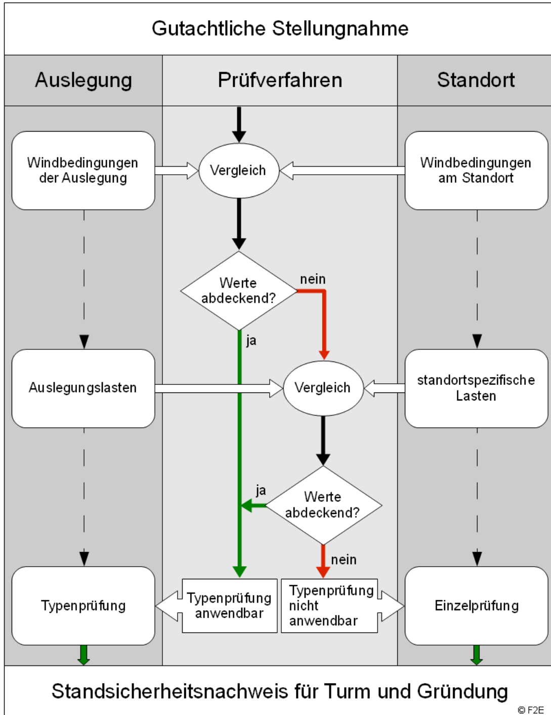
Abbildung 2.1.1: Schematische Darstellung des Prüfverfahrens.
