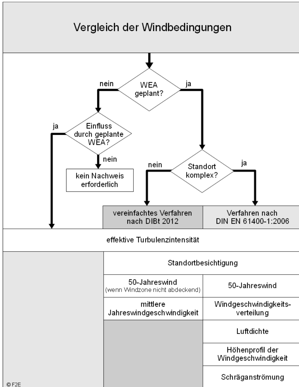
Abbildung 2.1.3: Nachweis durch Vergleich der Windbedingungen gemäß /2.8/.
