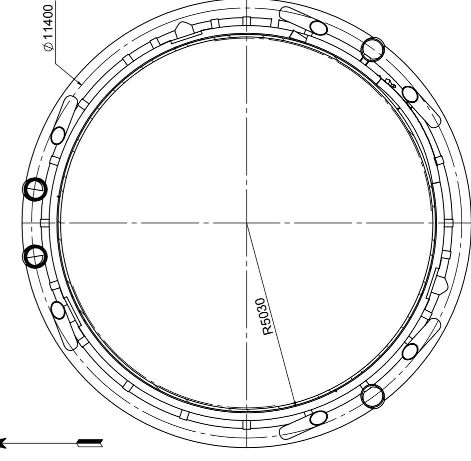
SEKTION C-C 1 : 100
