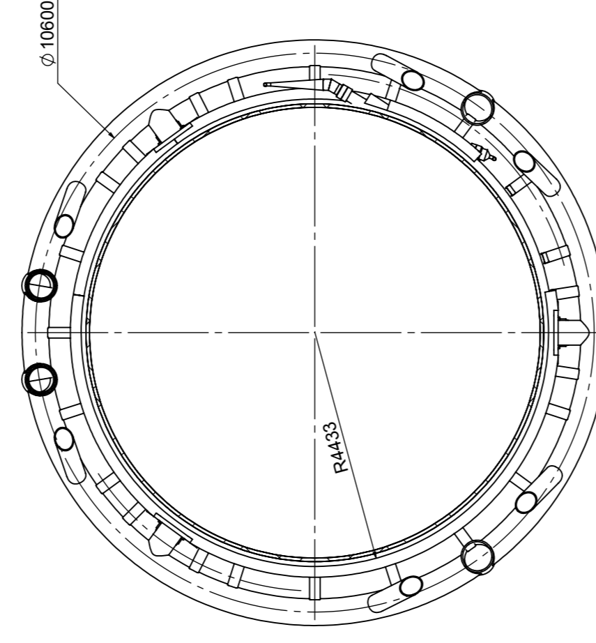
SEKTION B-B 1 : 100
