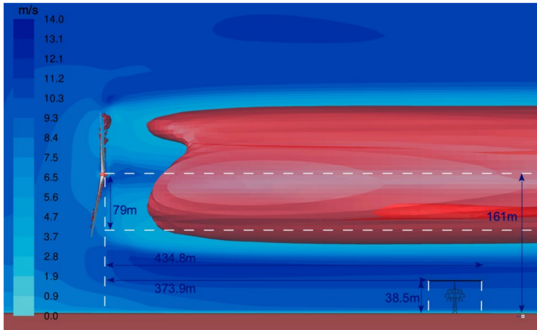
Abbildung 4.2.2.1: Vertikaler Schnitt in der Achse einer WEA vom Typ GE 5.5-158 5.5MW, NH 161.0m, bei einer Anströmung mit 10m/s. Dargestellt sind zusätzlich die Positionen der einzelnen Tragmasten der 380-kV-Leitung Güstrow - Parchim Süd entsprechend ihres Abstandes zu WEA 1 und 2. Weiterhin dargestellt ist der einhüllende Isoflächenbereich der auf 40% reduzierten Windgeschwindigkeit (rot).
