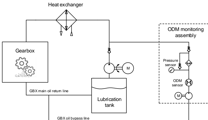
Abbildung 2: Ölpartikelsensor in das Getriebe-Schmiersystem integriert.
