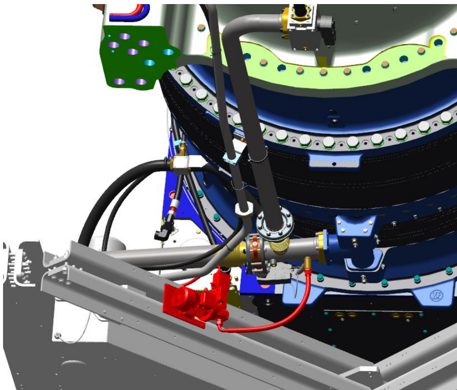
Abbildung 3. Darstellung der physischen Lage des ODM-Sensors.
