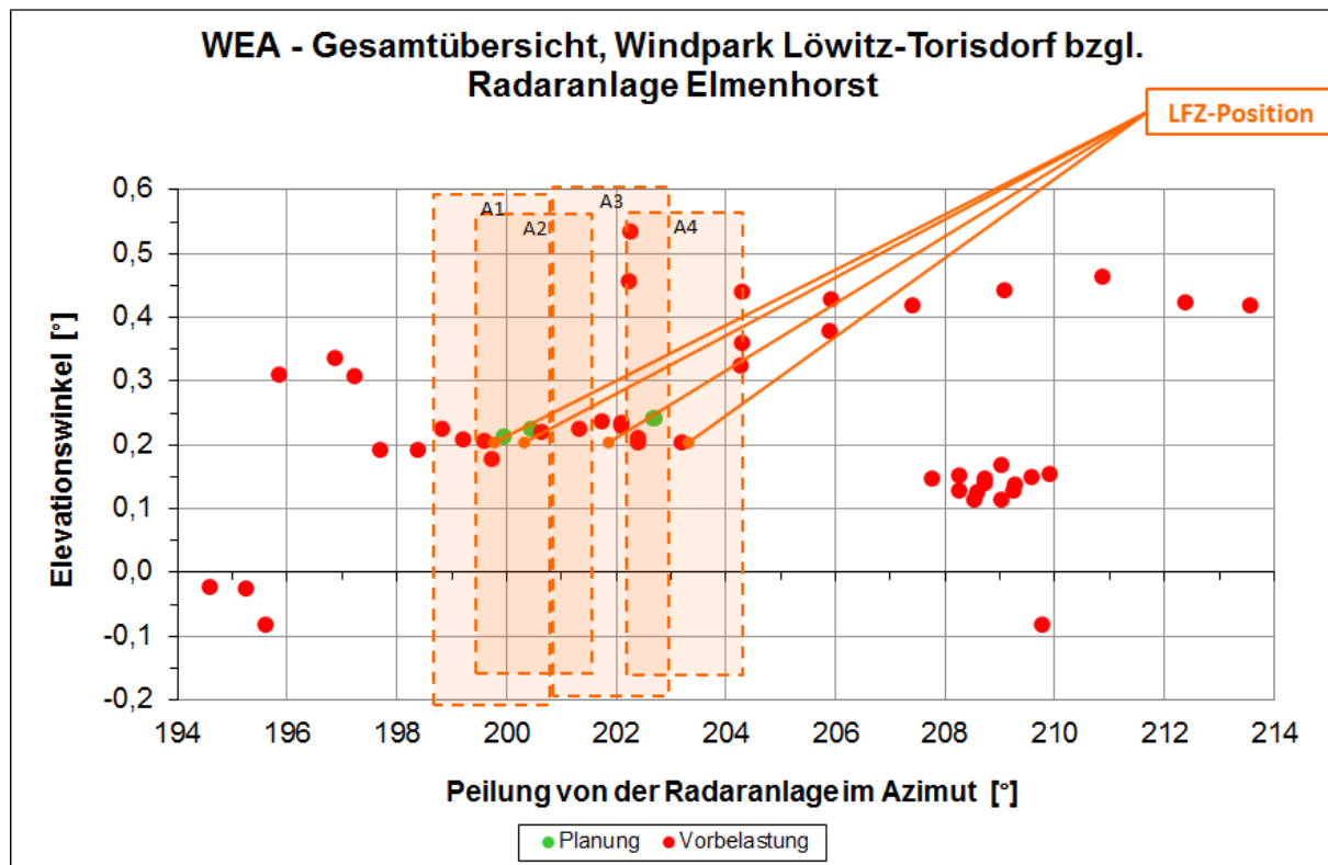
Abbildung 11: Perspektive zur Gondelanordnung gemäß Azimut und Elevation für die Position des Radars Elmenhorst. Die Bereiche der analysierten Teilanordnungen sind durch farbige Flächen gekennzeichnet. Die Richtung und Elevation des angenommenen Lfz ist dargestellt.
