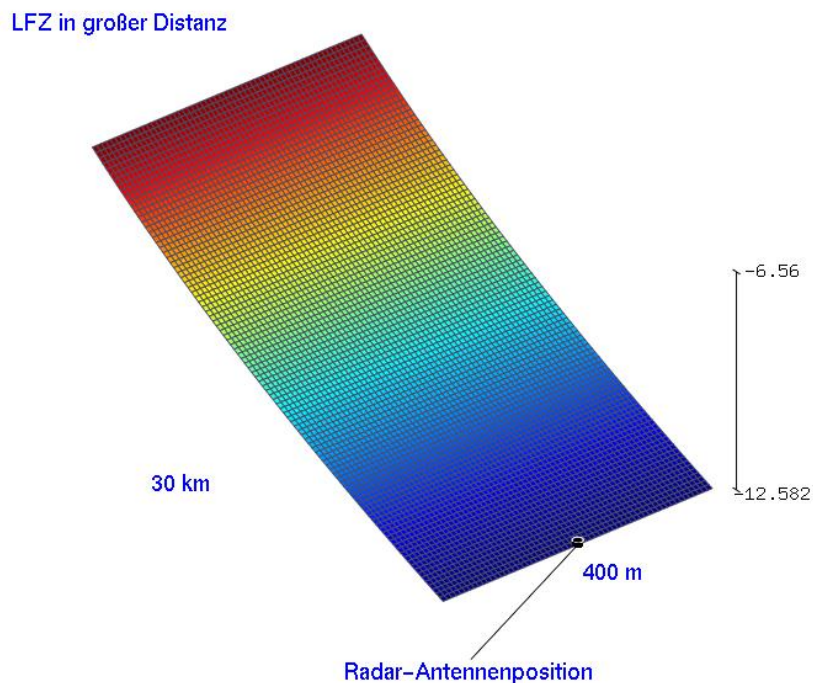
Abbildung 5: Das dargestellte Raumgebiet mit einer Elevation von 0,2° ohne WEA-Einfluss in der Konturdarstellung für die Betriebsfrequenz des Radars Elmenhorst
