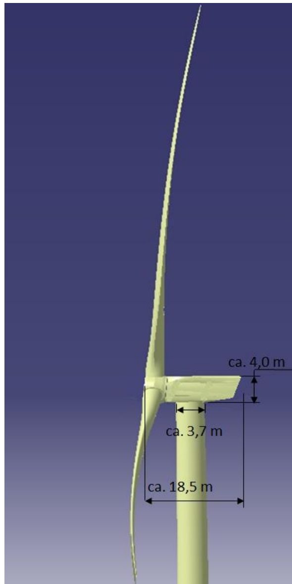
Abbildung 1: Schematische Objektgeometrie für die geplante WEA-Bauform Eno152-5.6 mit ca. 152 m Rotor
