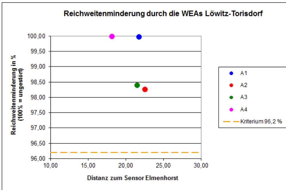
Abbildung 10: Übersicht über die zu erwartende Reichweitenreduktion bei den angegebenen WEA-Konstellationen.
