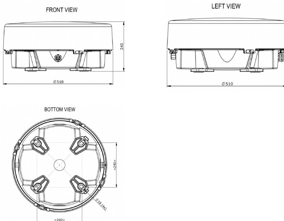
Abbildung 5-1: Gefahrenfeuer – Maße
