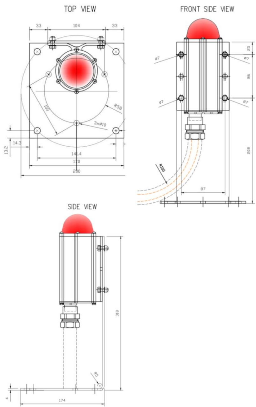
Abbildung 5-1 Abmessungen der Turmfeuer (LI-10-IR-DC)
