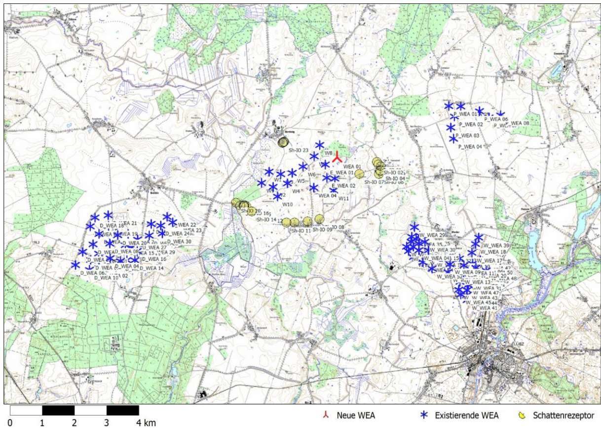
Abb. 1 Standorte der geplanten WEA, der existierenden WEA und der Immissionsorte
