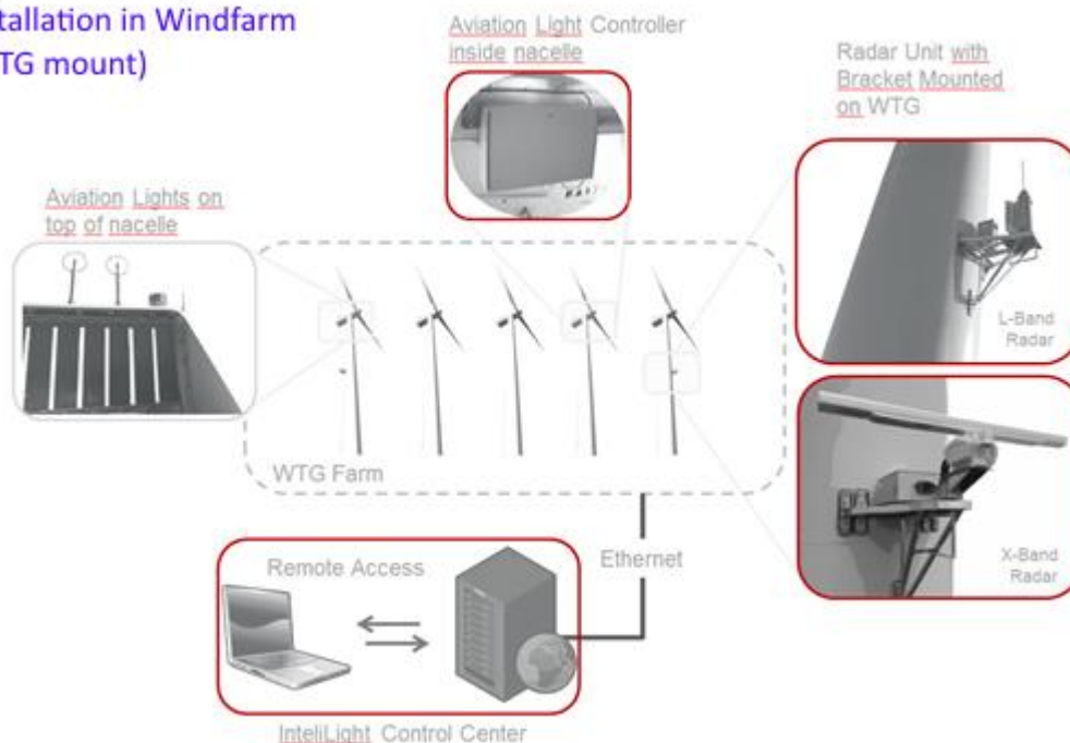
Abbildung 2-1: Darstellung der Systemkomponenten (rot gekennzeichnet). Oben: Flugbefeuerungssteuerungen. Rechts: X- und L-Band-Radare. Unten: IntelliLight Control Center.
