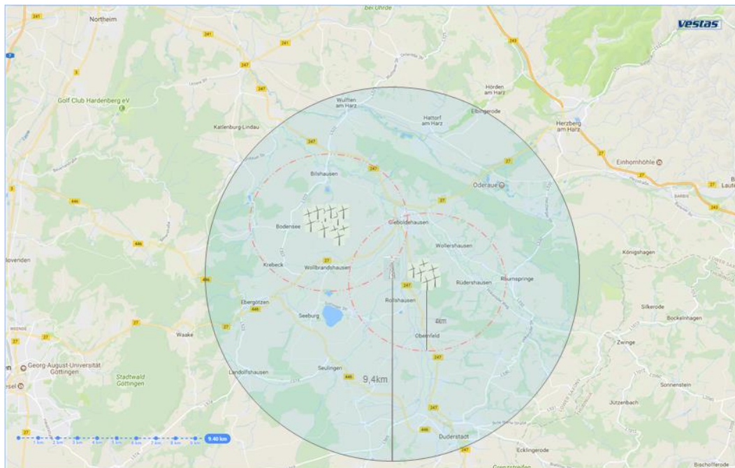
Abbildung 6-2: Abdeckung des Gebiets um die äußere Grenze der Windenergieanlage, wo das Radargerät auf einem externen Turm angebracht ist, durch das Vestas IntelliLight-Radar, im Beispiel gemäß der deutschen Vorschrift mit einer Warndistanz von 4 km.
