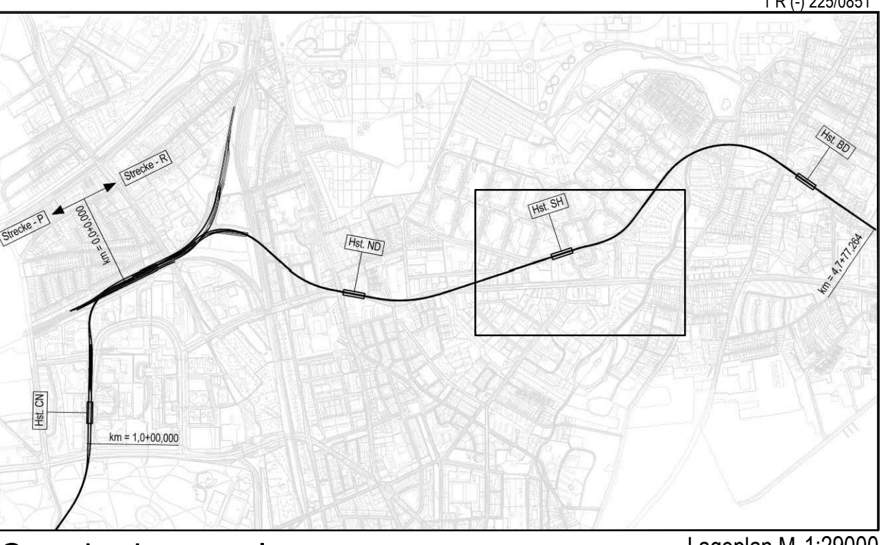
Genehmigungsplanung Lageplan M 1:20000
