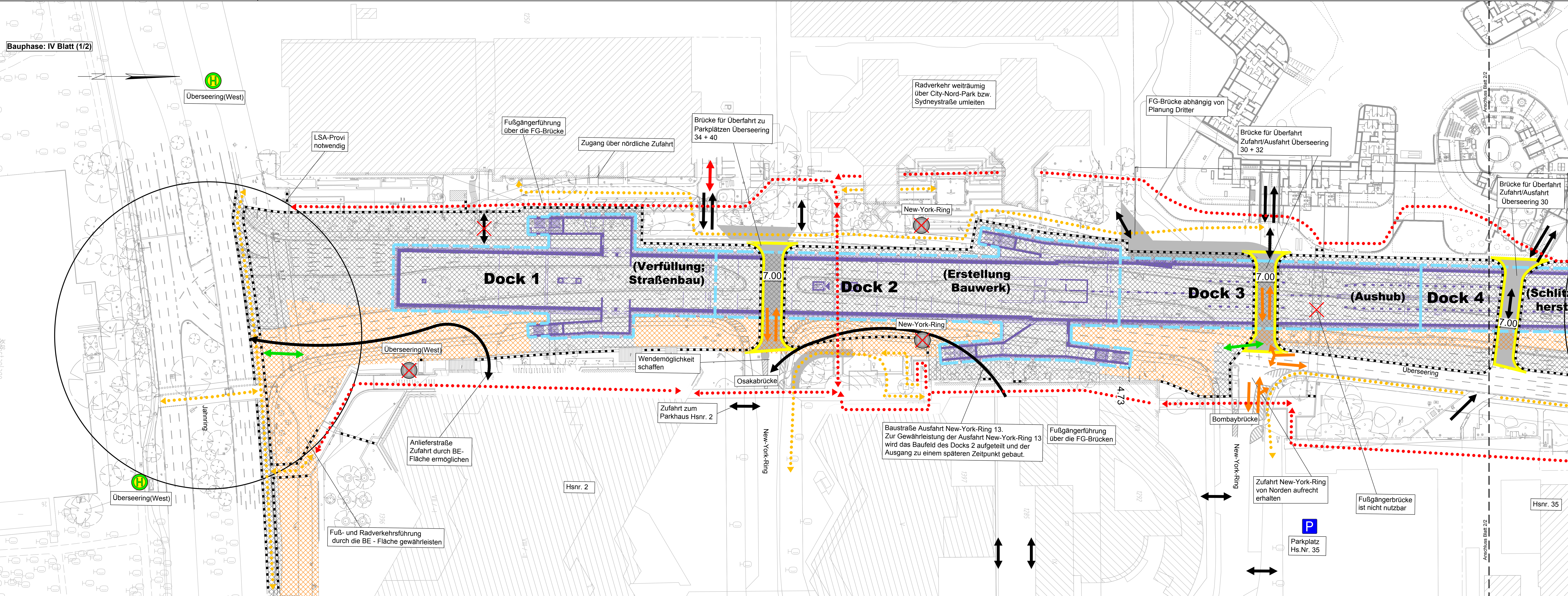
Genehmigungsplanung
