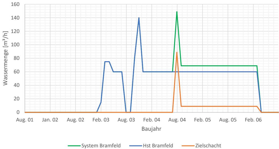
Abbildung 2: Maximaler Wasseranfall aus Leckagewasser und Lenzvorgängen in jedem Monat (ohne CGV-Arbeitsschacht)
