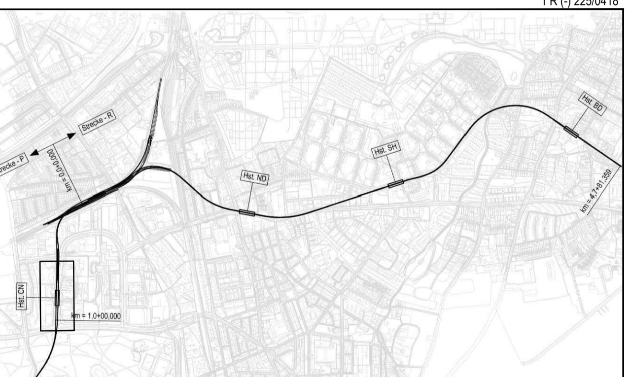
Genehmigungsplanung Lageplan M 1:29000
