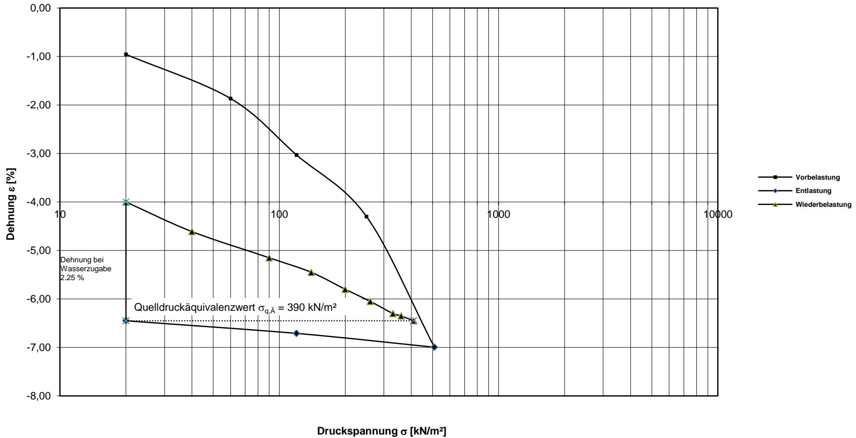
Spannungs-Verformungsdiagramm
