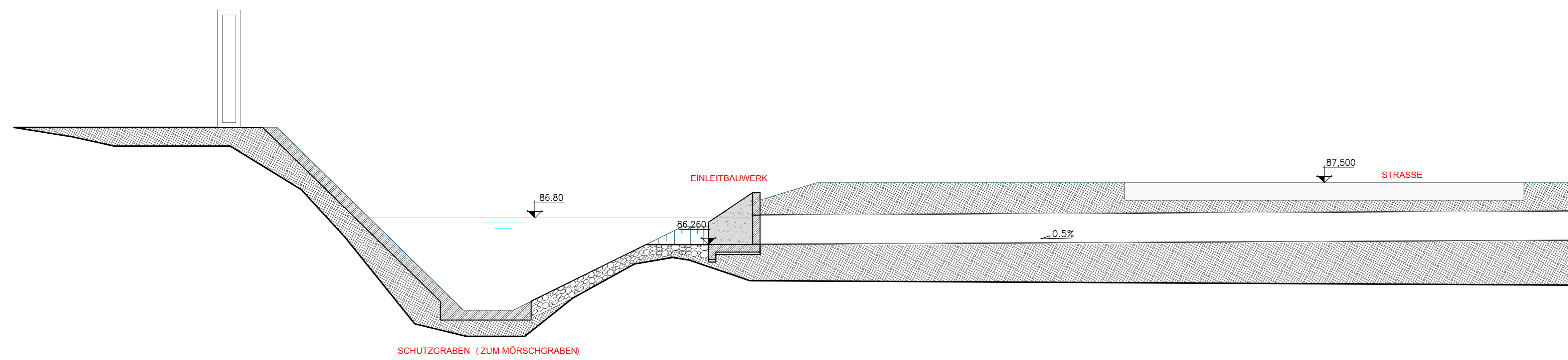
DETAIL 1 MASSTAB: 1:50 GRAFISCHER MASSTAB IN METERN
