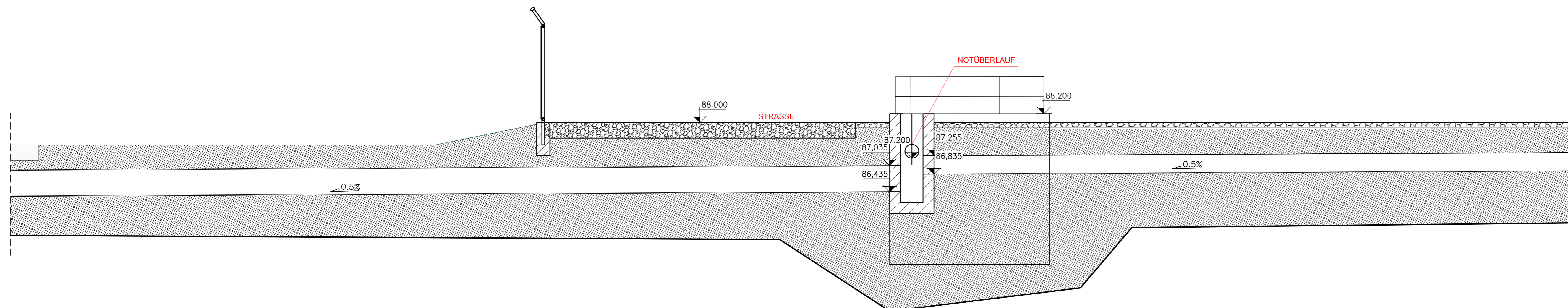
DETAIL 2 MASSTAB: 1:50 GRAFISCHER MASSTAB IN METERN
