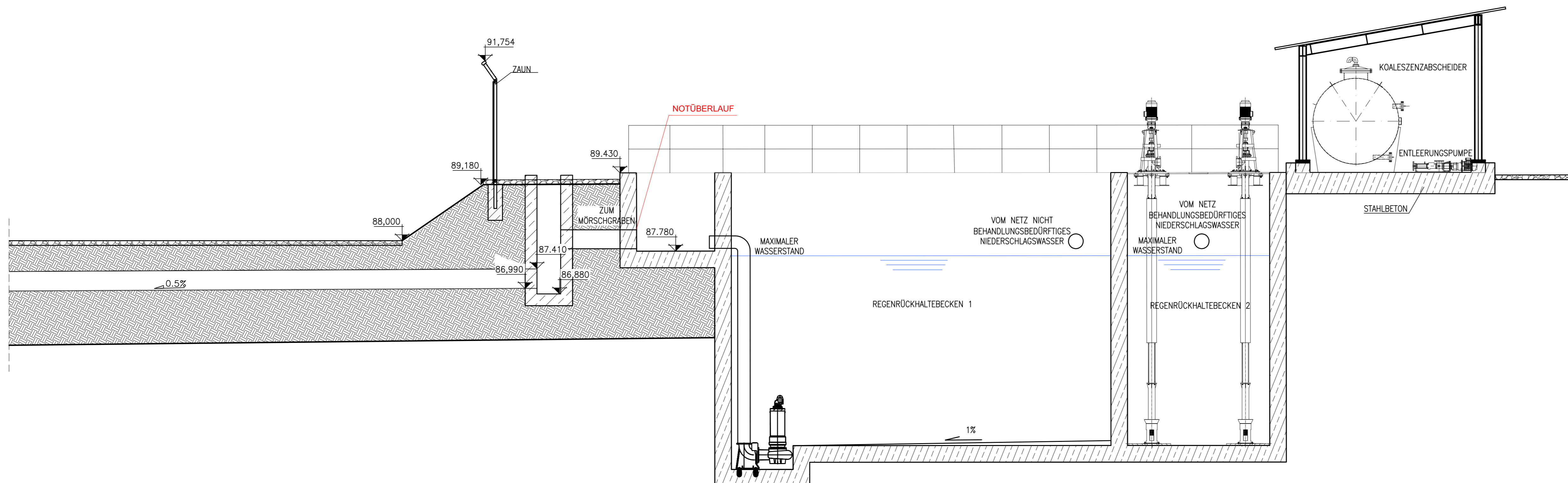
DETAIL 3 MASSTAB: 1:50 GRAFISCHER MASSTAB IN METERN
