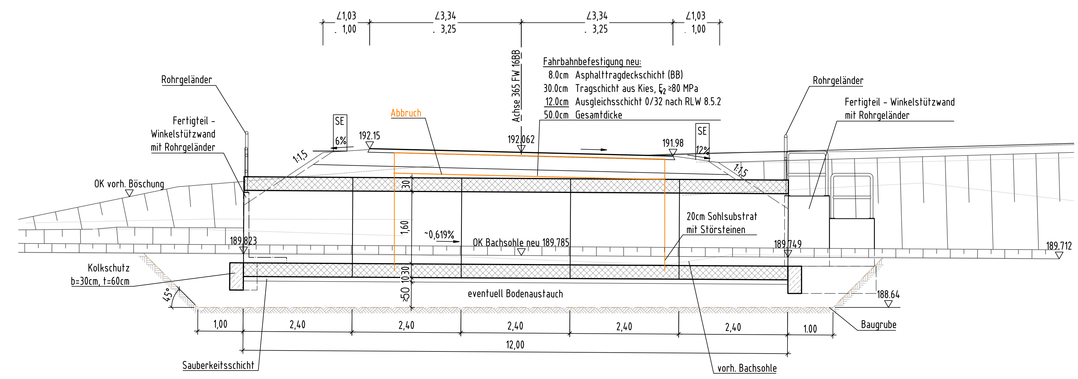
Regelquerschnitt RQ-RQ M 1:50 Station 0+027.345
