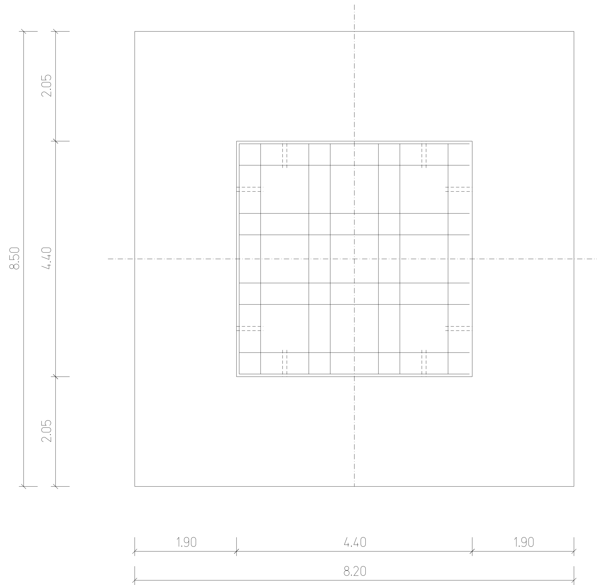
Grundriss
