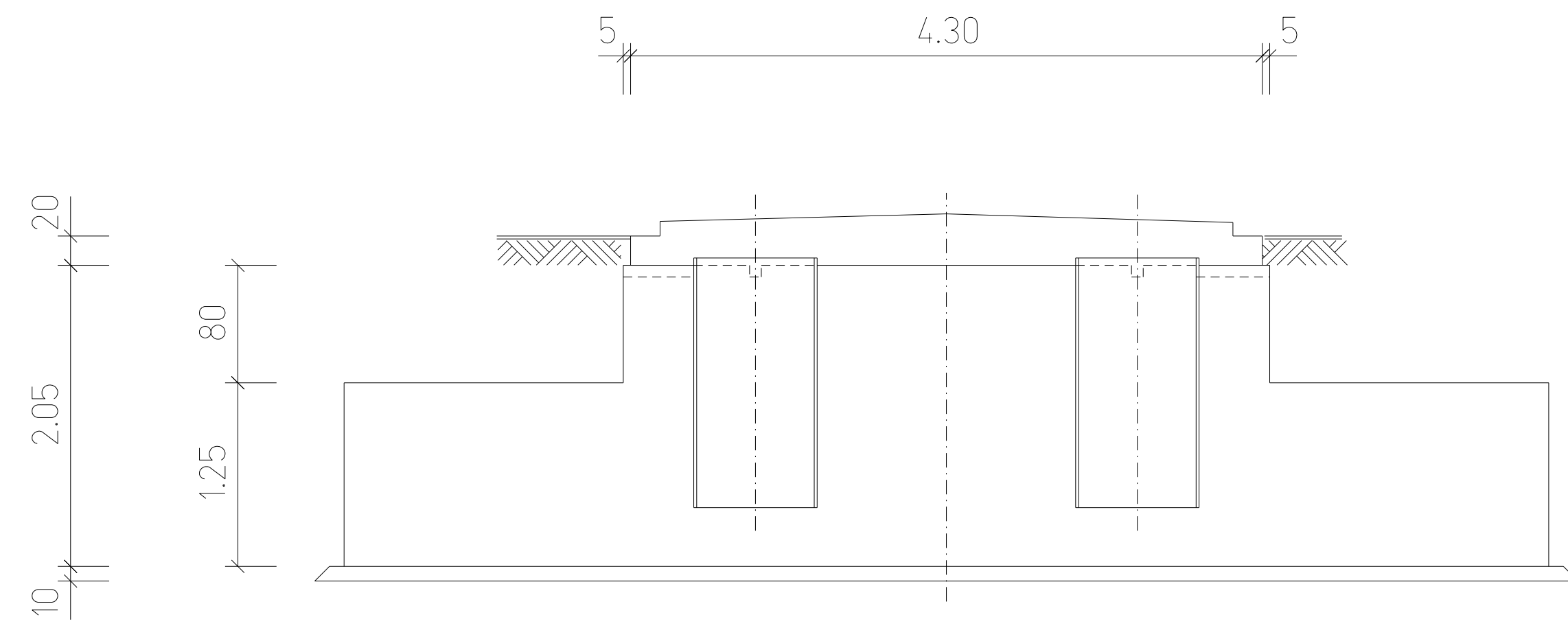
Längsschnitt
