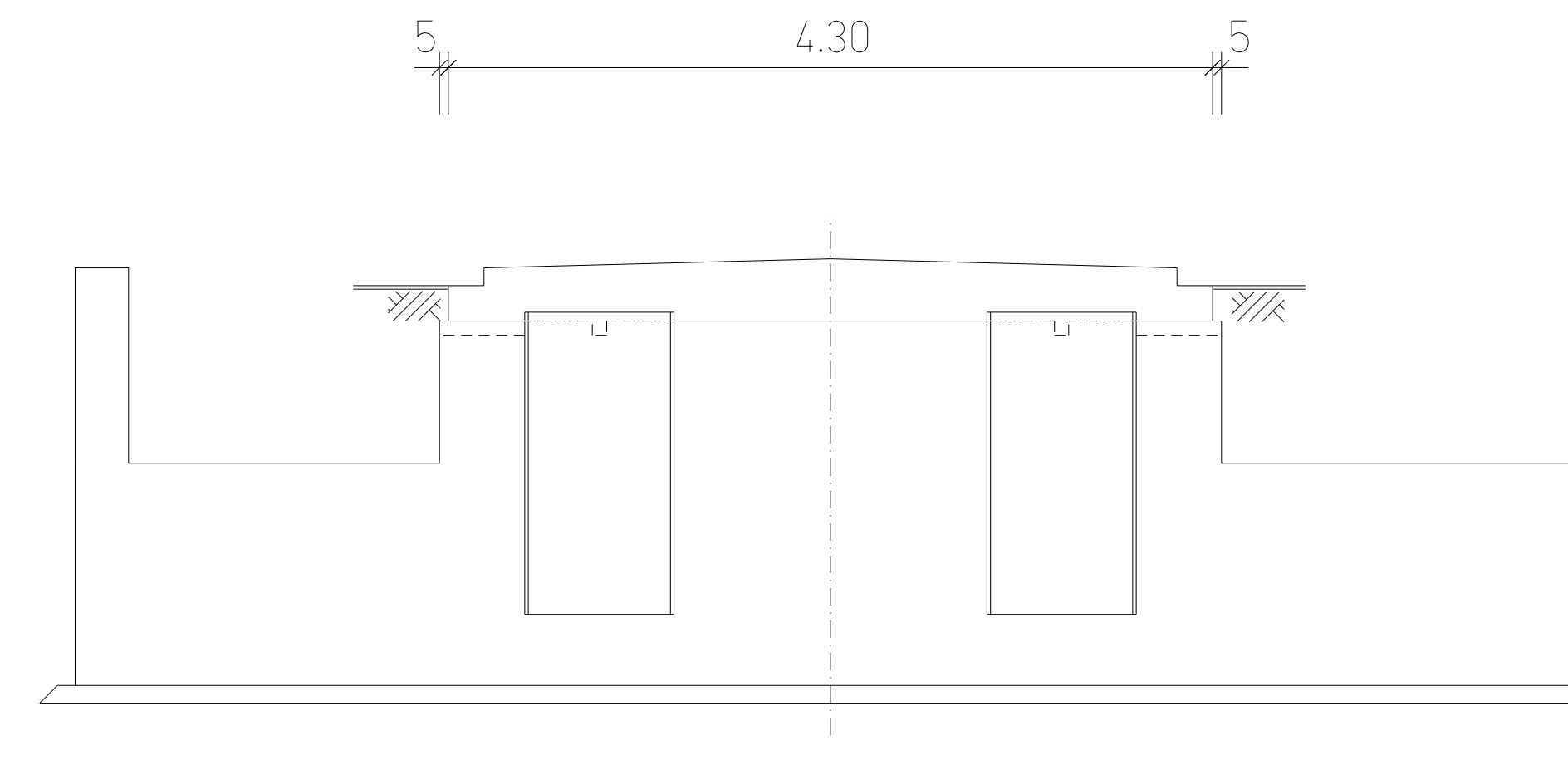
Querschnitt
