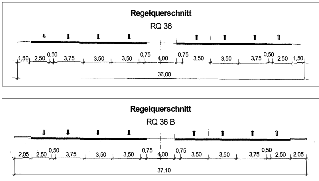
Abb. 4 : Regelquerschnitte Strecke und Bauwerk
