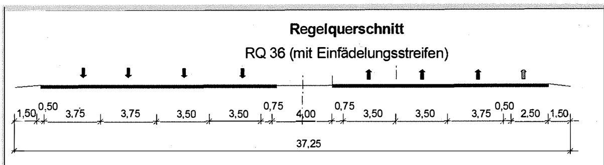
Abb. 8 geplanter Streckenregelquerschnitt RQ 36 mit Einfädelungstreifen von Bau-km 2+820 bis Bauende
