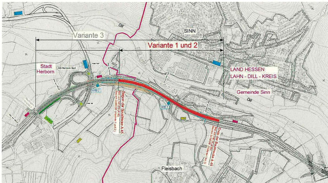
Abb. 5 : Übersichtslageplan mit Darstellung der Varianten
