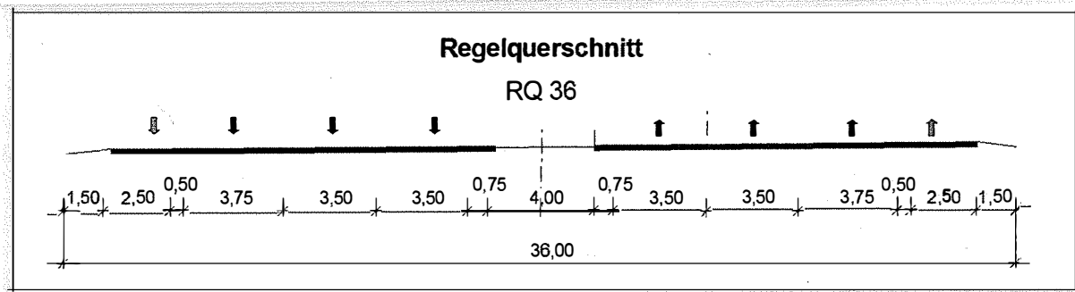
Abb. 7 geplanter Streckenregelquerschnitt RQ 36
