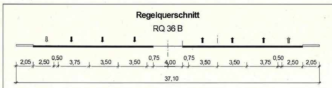
Abb. 6 geplanter Brückenregelquerschnitt RQ 36 B
