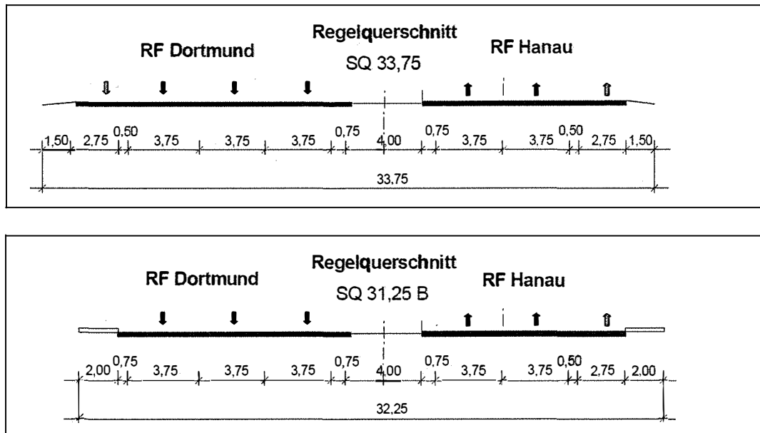
Abb. 3 : Vorhandene Regelquerschnitte Strecke (SQ 33,75) und Bauwerk (SQ 31,25B)
