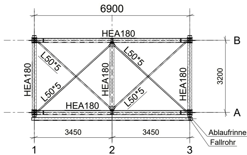
Draufsicht Dach 22 - Stahlbau 1:100
