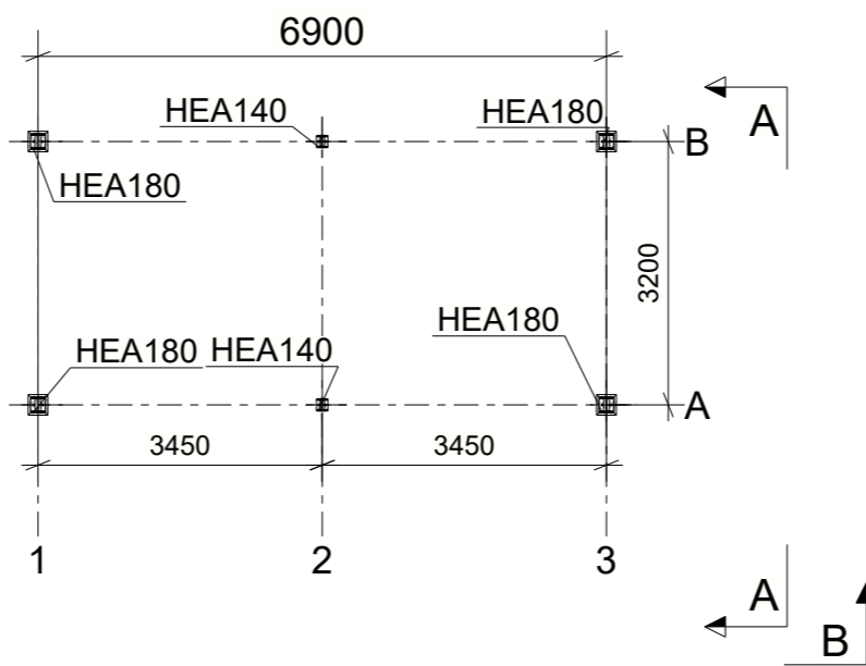
Draufsicht Dach 22 - Fussplatten 1:100
