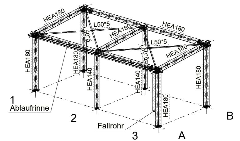
3D Perspektive Stahlbau 1:100
