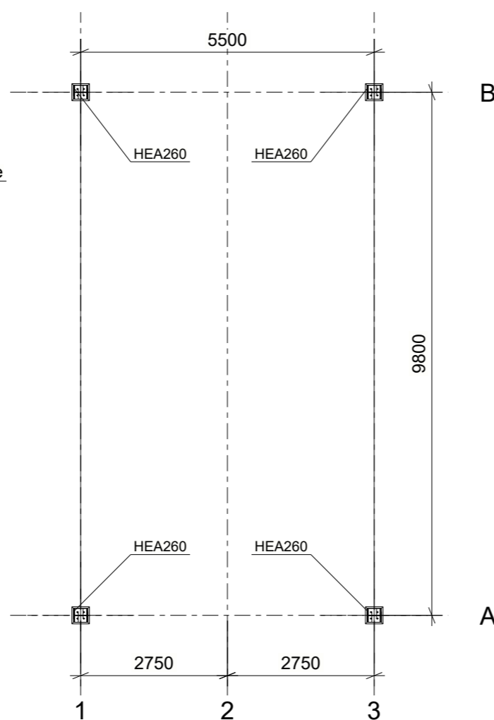
Draufsicht Dach Nr.21 - Fussplatten 1:100
