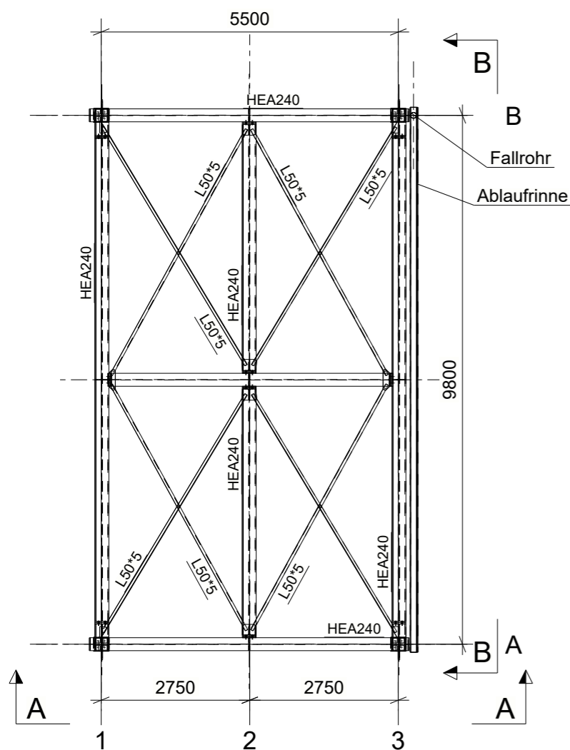
Draufsicht Dach Nr.21 - Stahlbau 1:100
