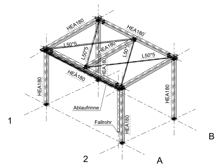
3D Perspektive Stahlbau 1:100
