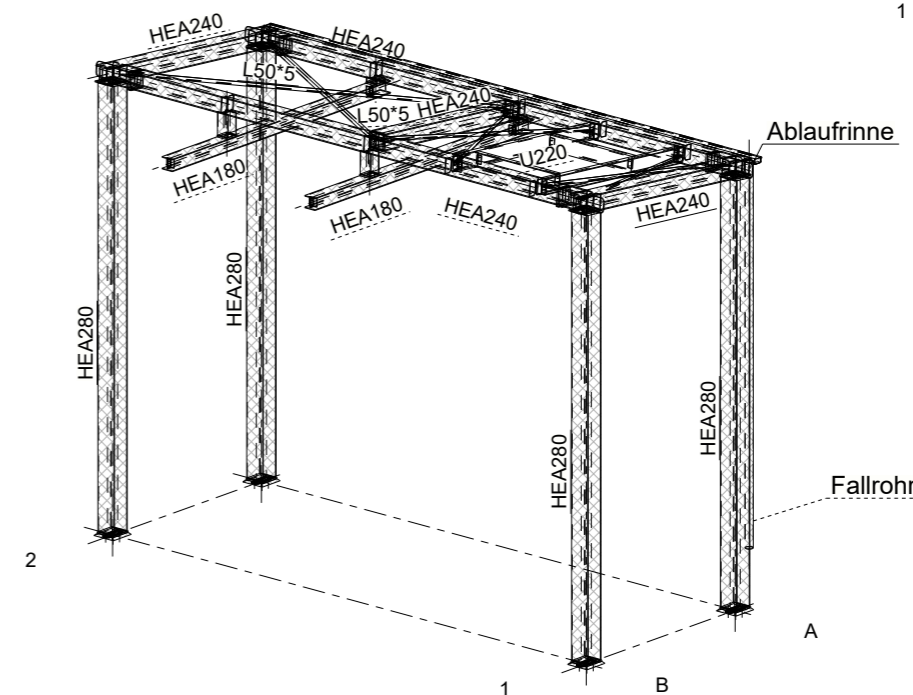
Draufsicht Dach 3AB - komplett 1:100
