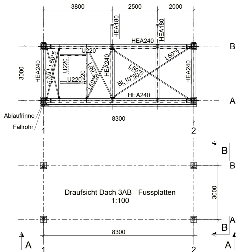
Draufsicht Stahbau Dach 3AB 1:100
