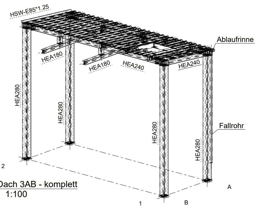
Draufsicht Dach 3AB - komplett 1:100
