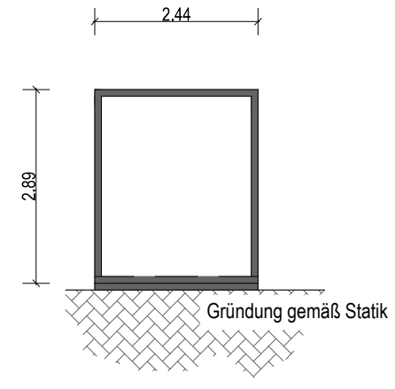
Schnitt A-A
