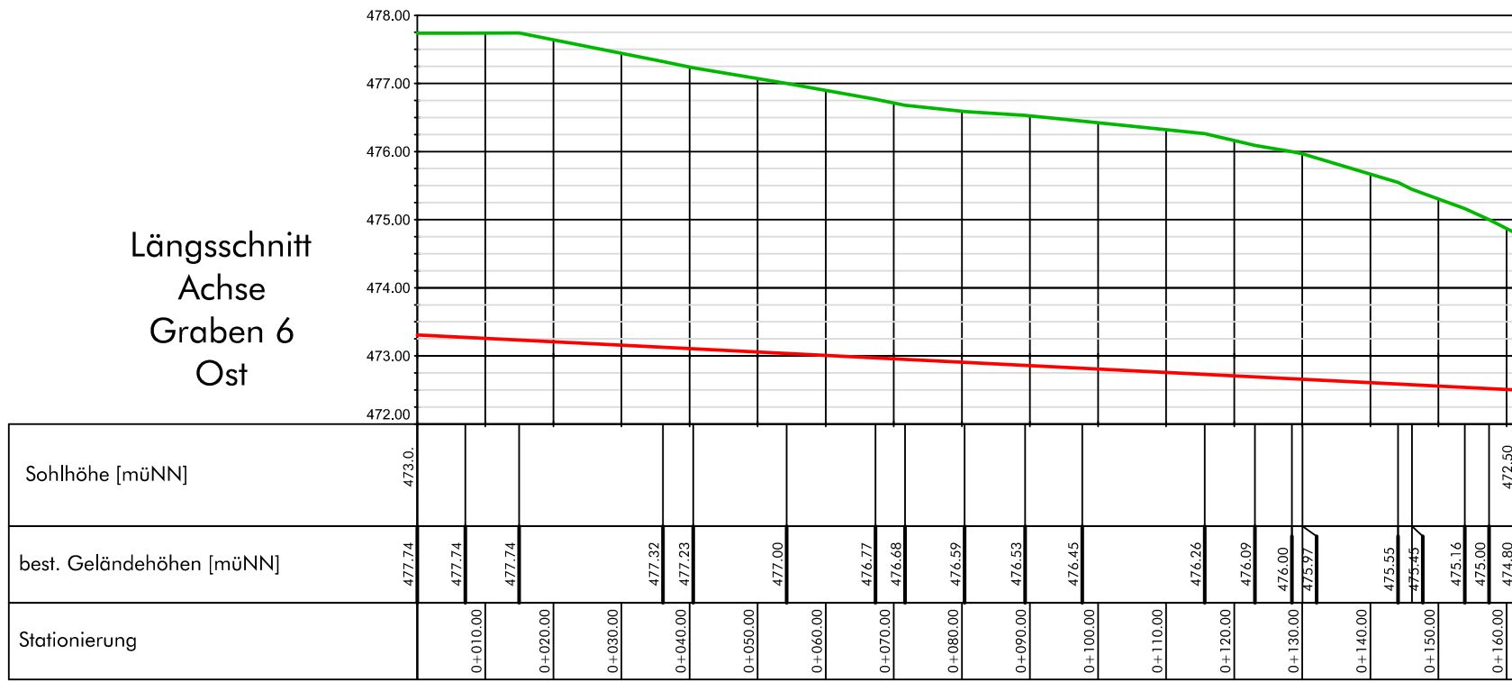
Längsschnitt Achse Graben 7 Süd
