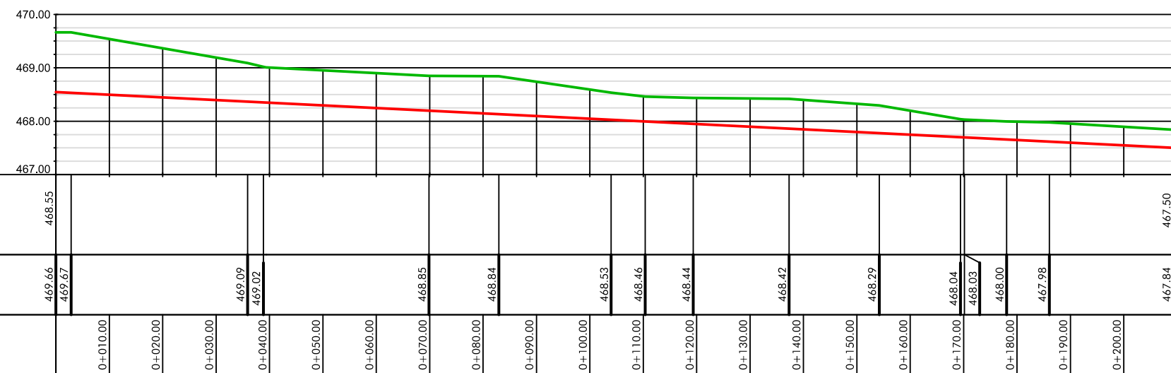
Längsschnitt Achse Graben 3 N nord
