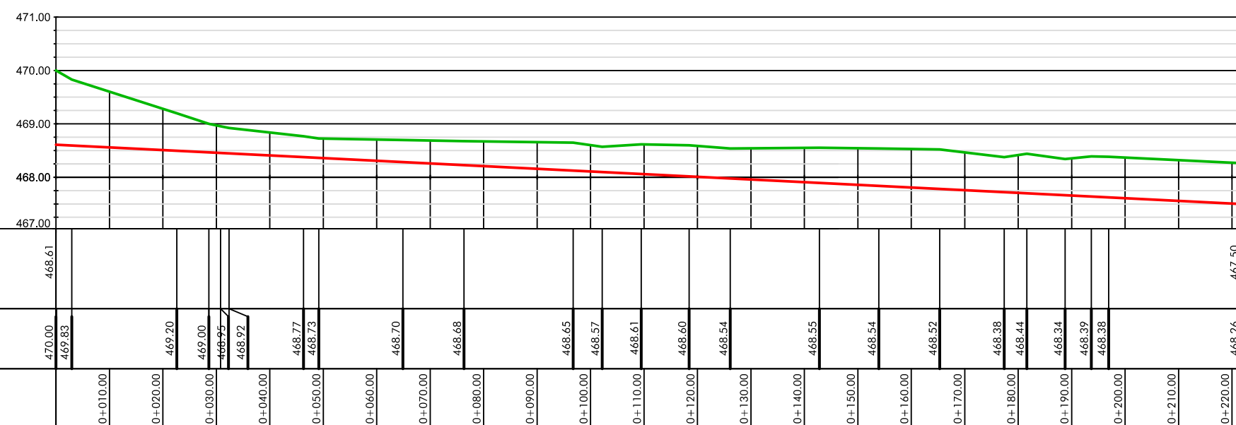
Längsschnitt Achse Graben 4 Nord
