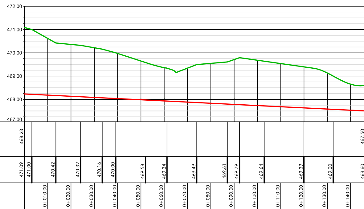
Längsschnitt Achse Graben 2 Bestand
