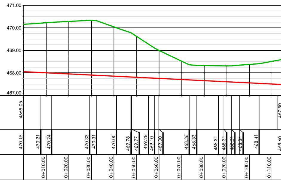
Längsschnitt Achse Graben 1 Bestand
