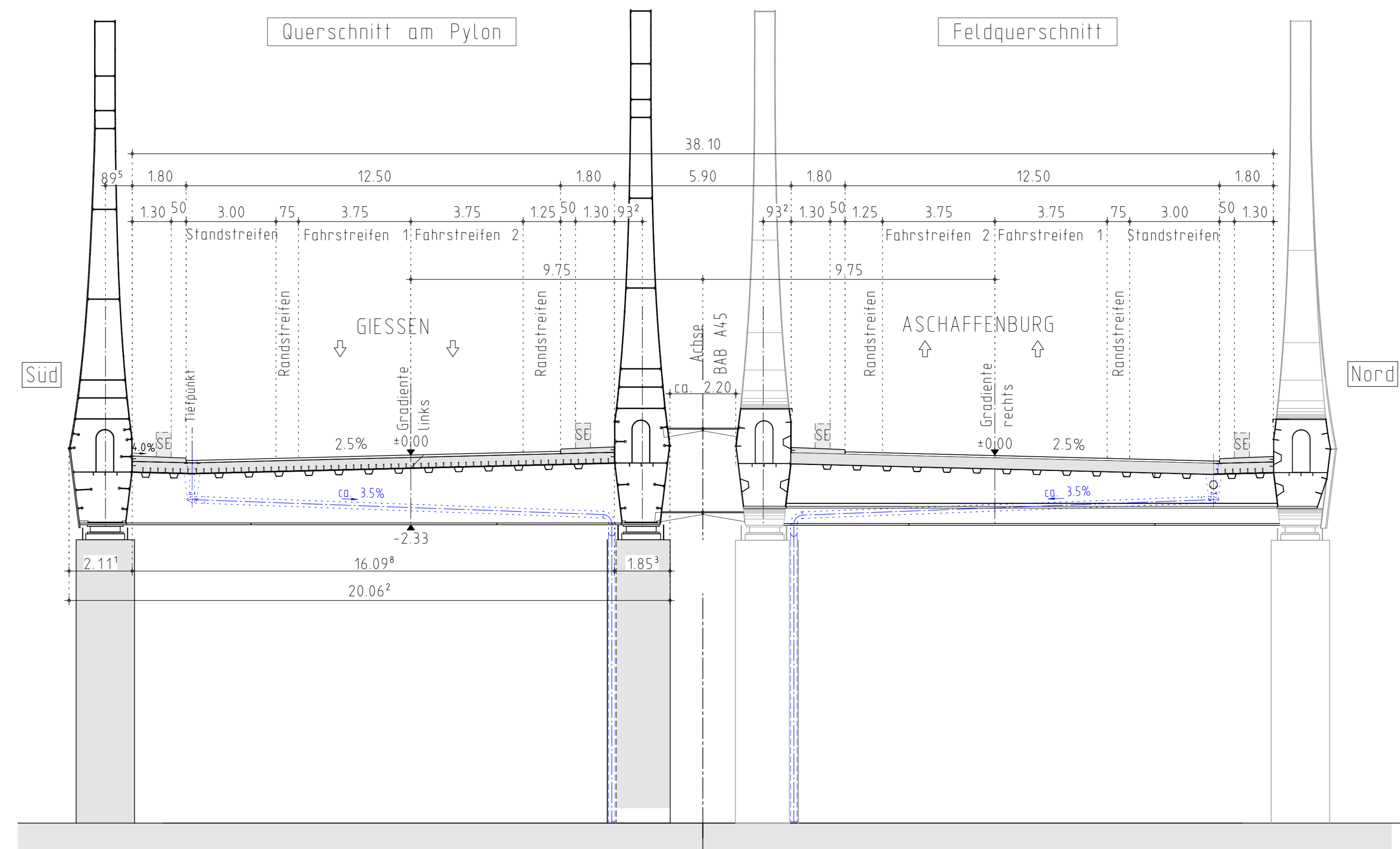
Querschnitt Strombrücke 1:100
