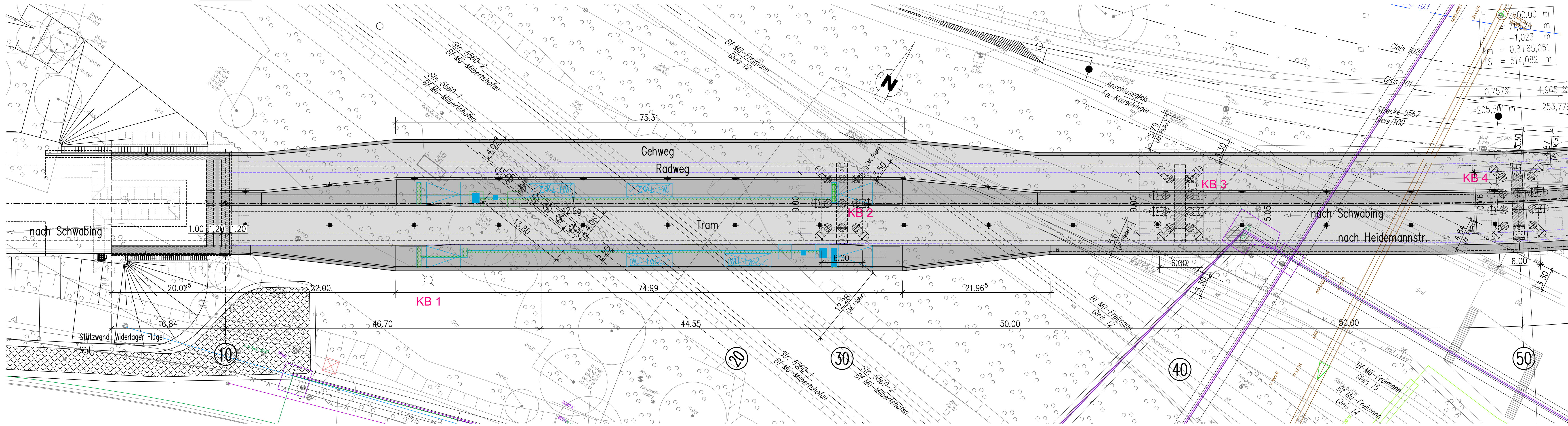
Grundriß M 1:250
