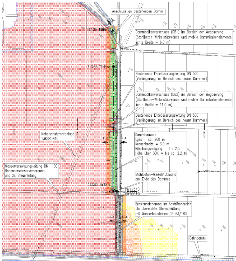
Abb. 2: Ausschnitt aus der Vorplanung zu Variante 2 Ingenieurbüro Winkler und Partner GmbH Stand 13.04.16
