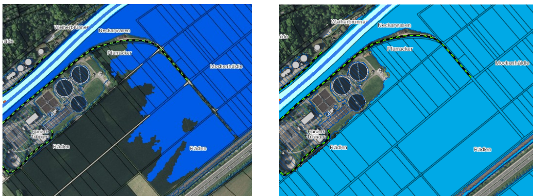
Abb. 7: Überflutungsflächen HQ_{10} (links) und HQ_{50} (rechts)
