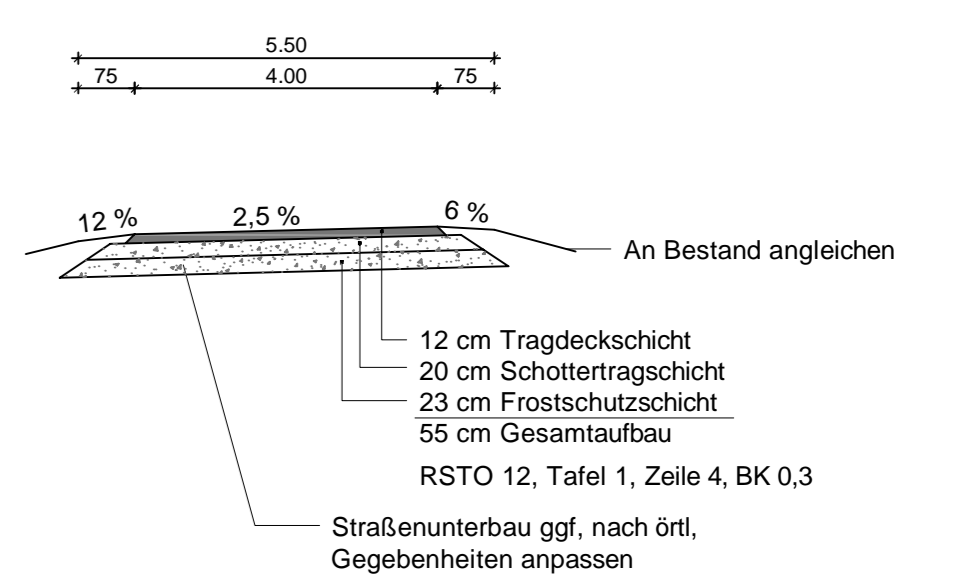
Regelaufbau Wirtschaftsweg Nordumfahrung M 1:100
