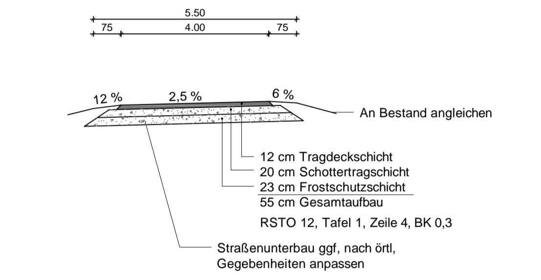
Regelaufbau Wirtschaftsweg Nordumfahrung M 1:100
