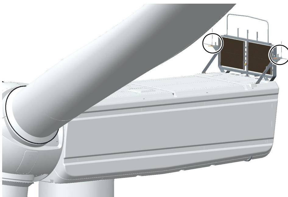
Abb. 1 Verbauposition der Gefahrenfeuer bei Delta4000
