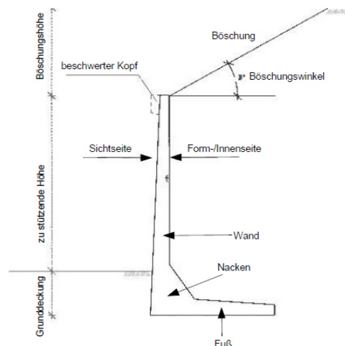
Abb. 2 Hangbelastete Fußseite
