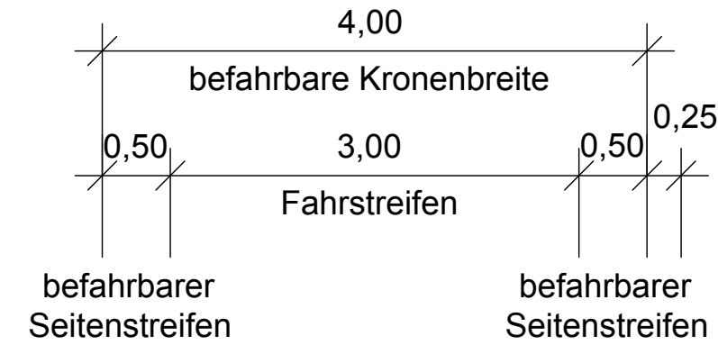
Wirtschaftsweg mit Asphaltdecke
