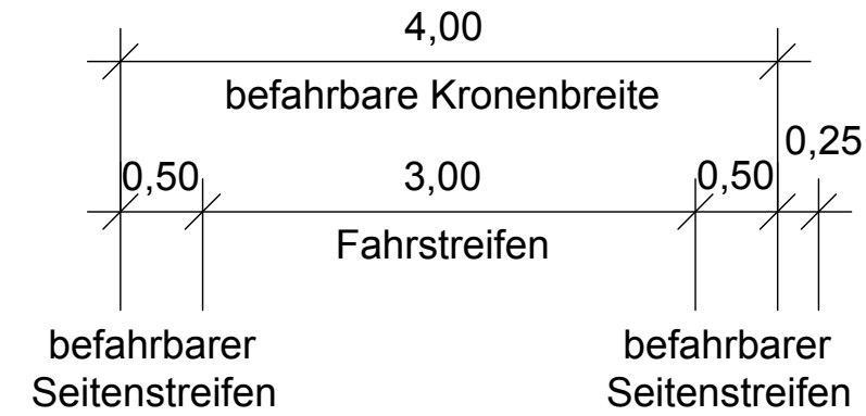
Wirtschaftsweg mit ungebundener Fahrbahndecke
