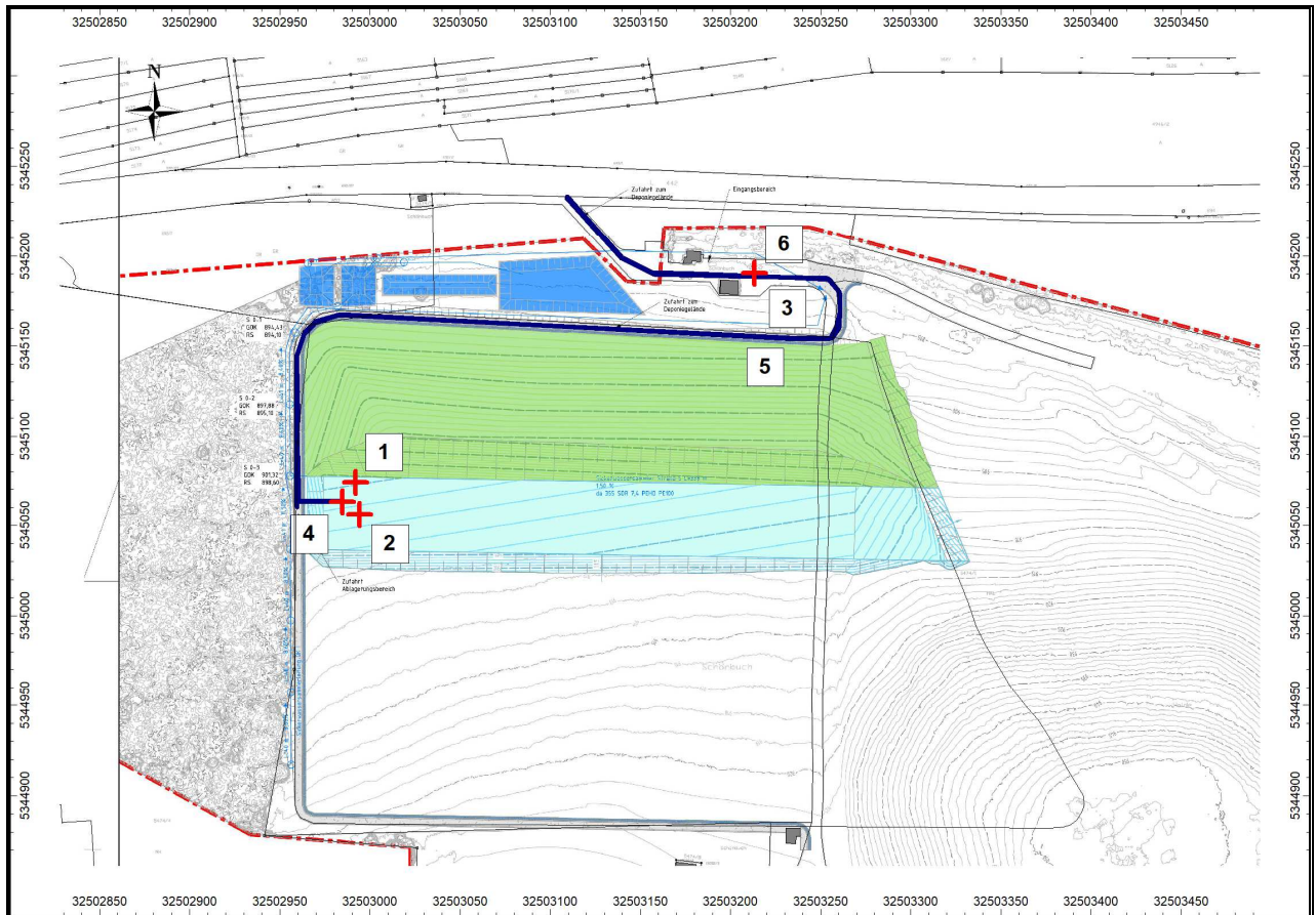
Abb. 8: Lage der Quellen Betriebsabschnitt BA 0.3 – IO1
