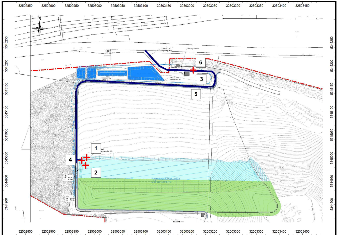
Abb. 14: Lage der Quellen Betriebsabschnitt BA 1.2 – IO1
