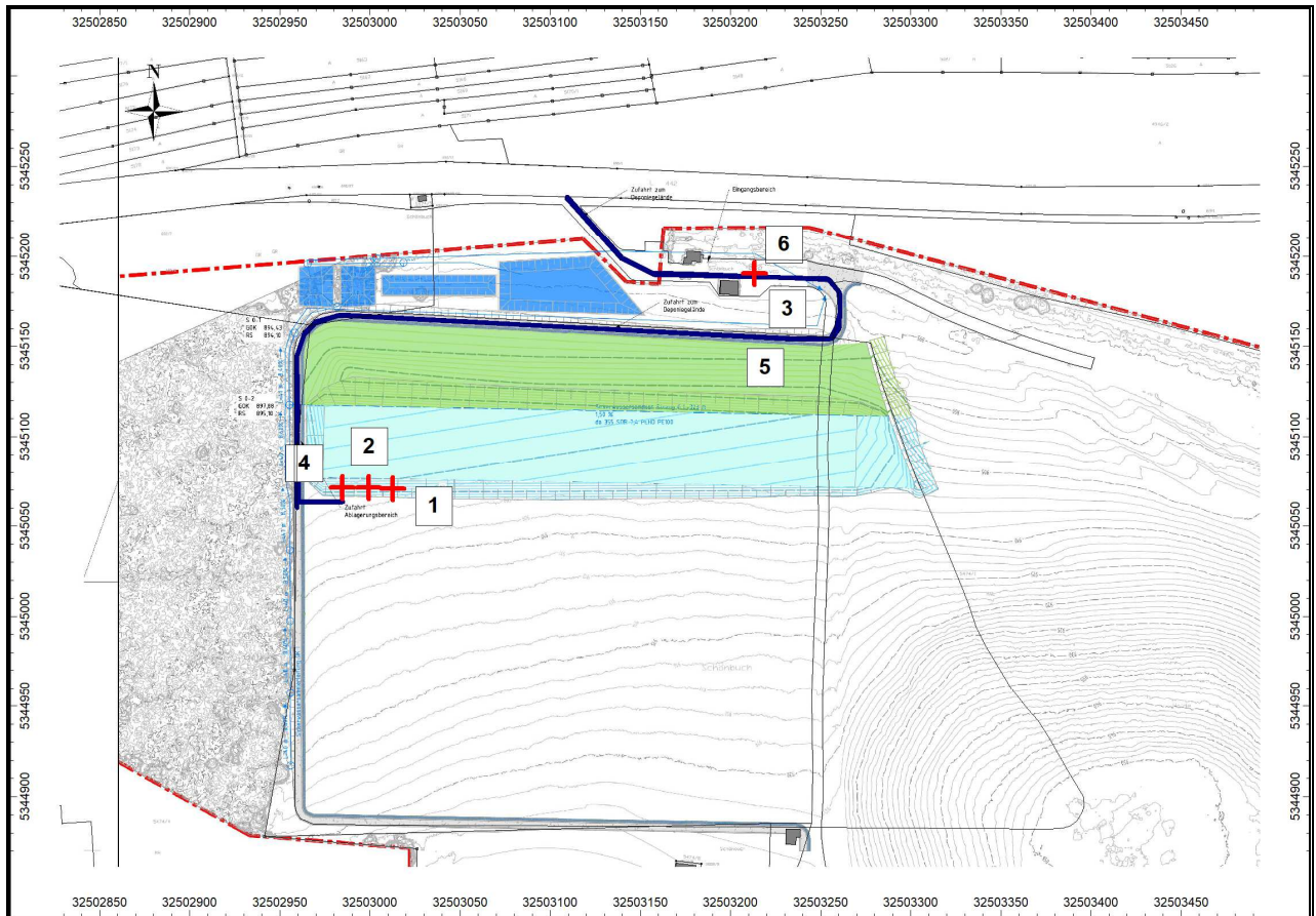
Abb. 7: Lage der Quellen Betriebsabschnitt BA 0.2 – IO3
