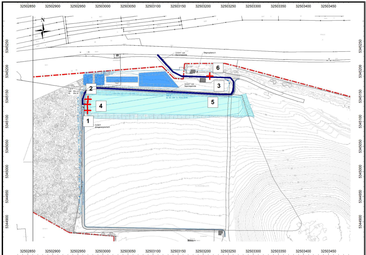
Abb. 3: Lage der Quellen Betriebsabschnitt BA 0.1 – IO2
