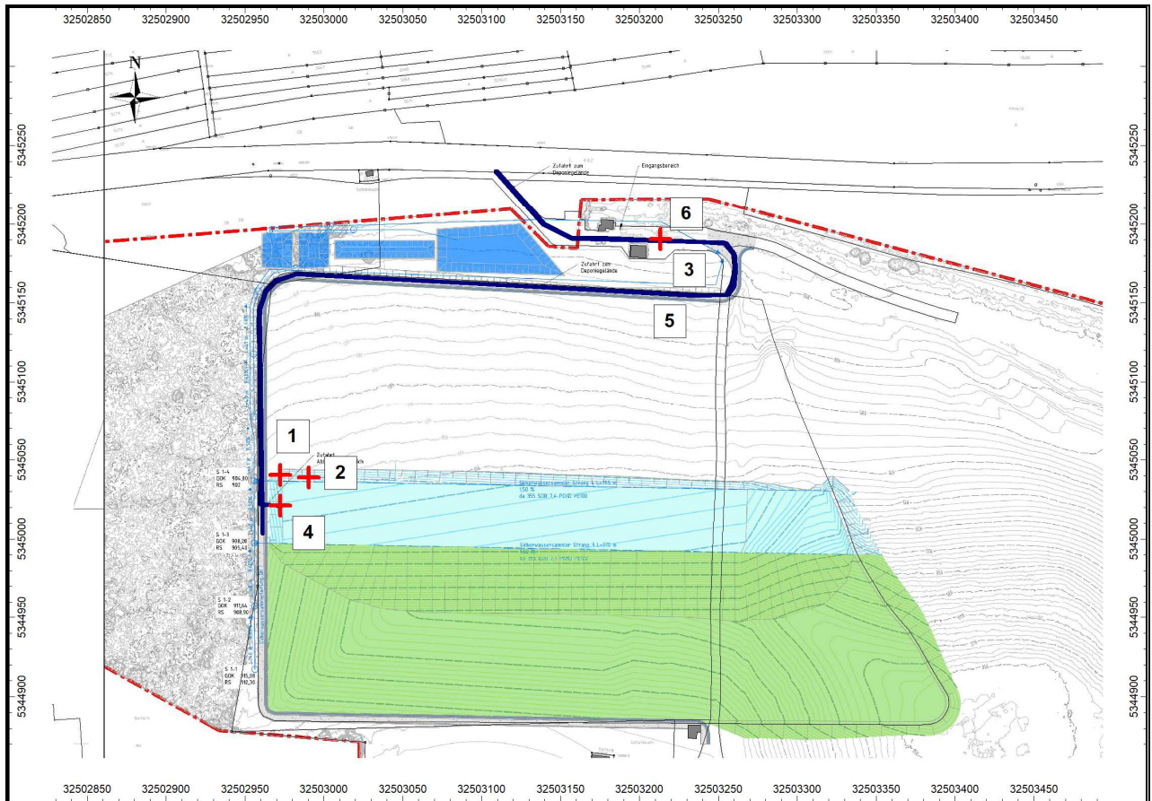
Abb. 17: Lage der Quellen Betriebsabschnitt BA 1.3 – IO1
