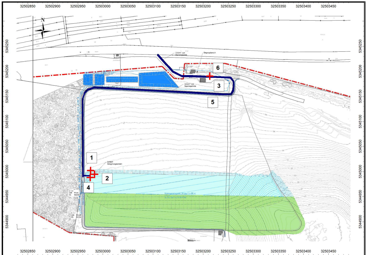
Abb. 15: Lage der Quellen Betriebsabschnitt BA 1.2 – IO2
