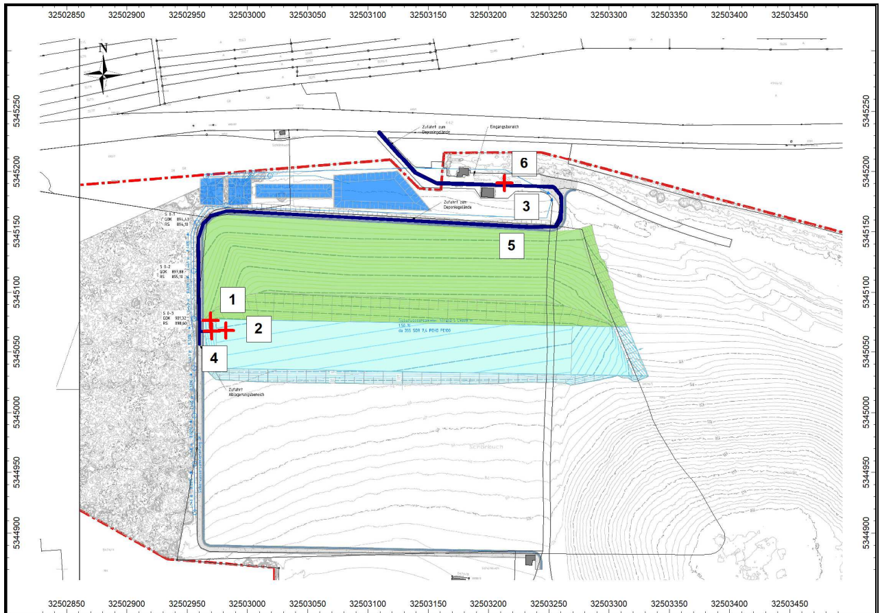
Abb. 9: Lage der Quellen Betriebsabschnitt BA 0.3 – IO2
