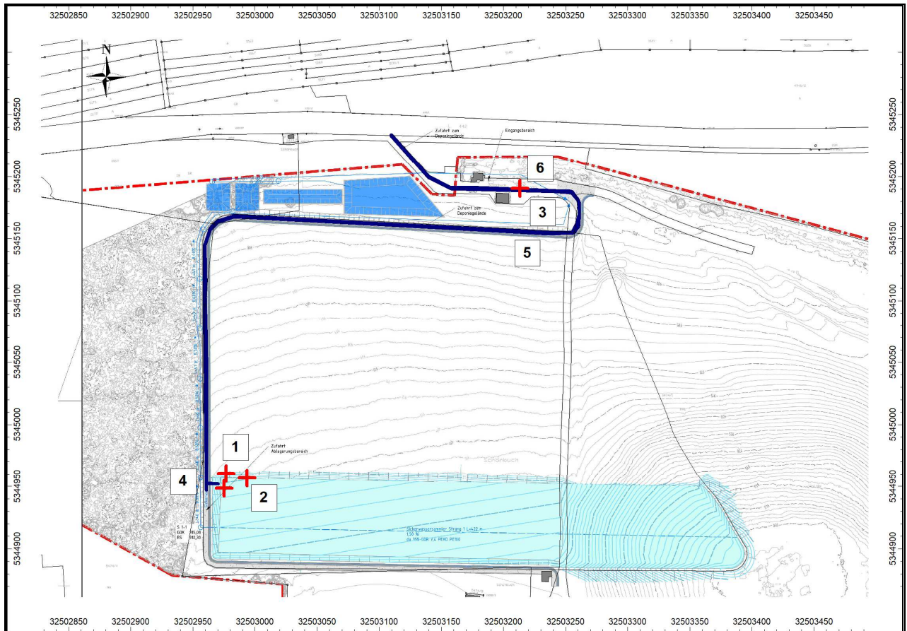
Abb. 11: Lage der Quellen Betriebsabschnitt BA 1.1 – IO1
