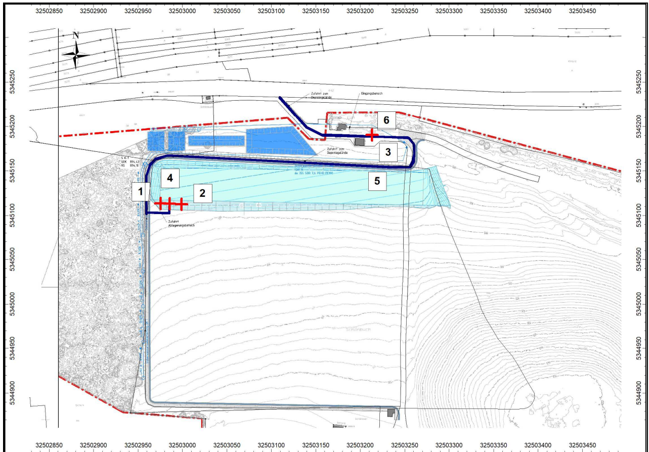
Abb. 4: Lage der Quellen Betriebsabschnitt BA 0.1 – IO3
