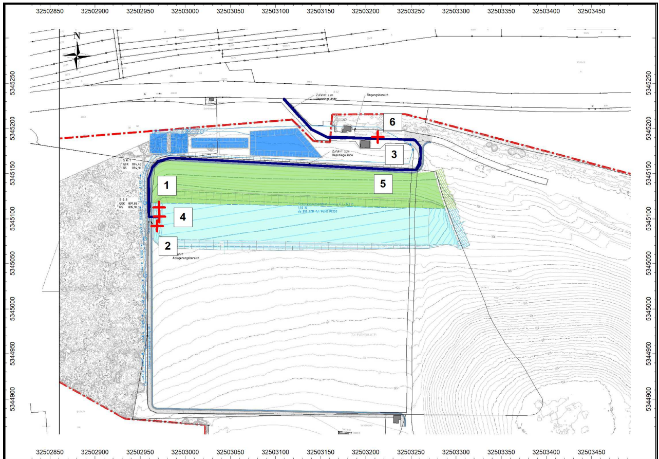
Abb. 6: Lage der Quellen Betriebsabschnitt BA 0.2 – IO2
