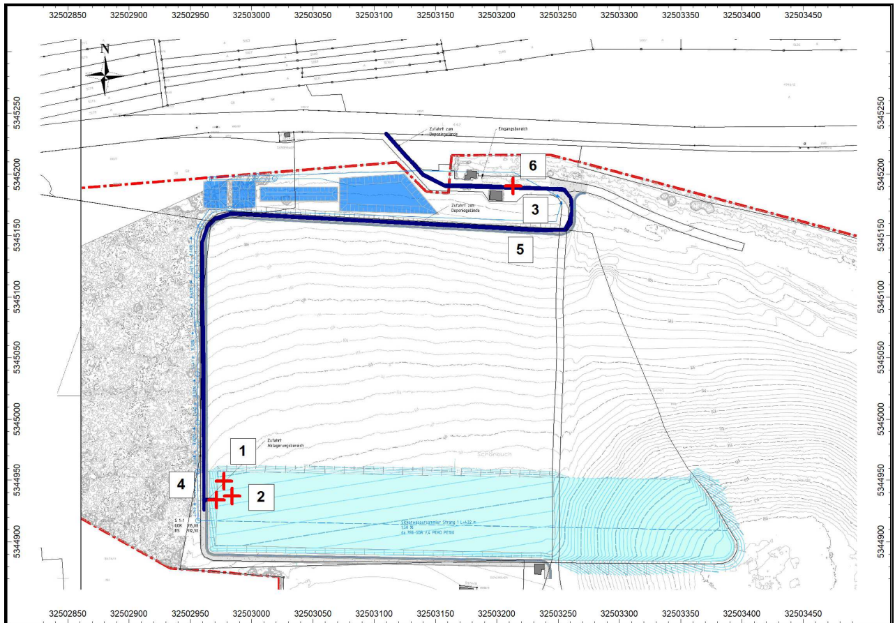
Abb. 13: Lage der Quellen Betriebsabschnitt BA 1.1 – IO3
