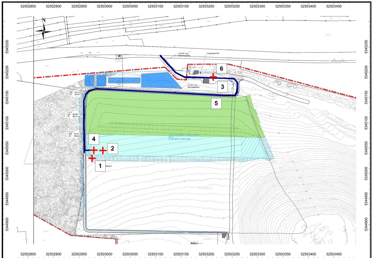
Abb. 10: Lage der Quellen Betriebsabschnitt BA 0.3 – IO3
