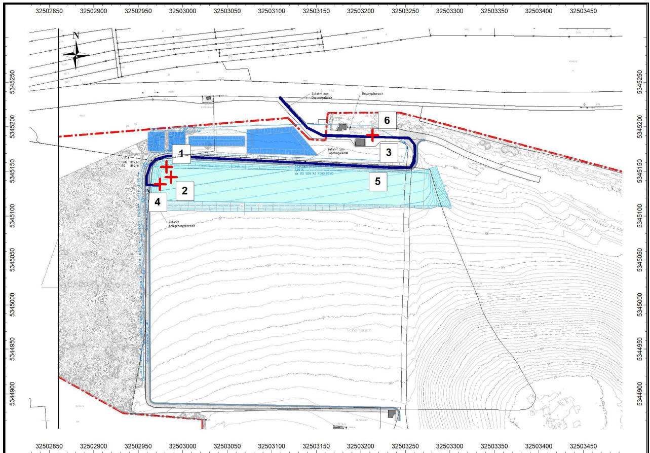
Abb. 2: Lage der Quellen Betriebsabschnitt BA 0.1 – IO1
