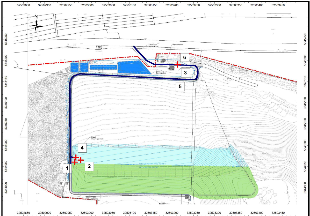
Abb. 16: Lage der Quellen Betriebsabschnitt BA 1.2 – IO3
