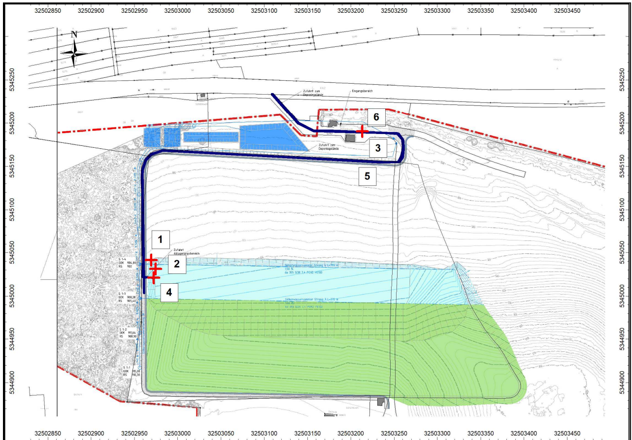
Abb. 18: Lage der Quellen Betriebsabschnitt BA 1.3 – IO2
