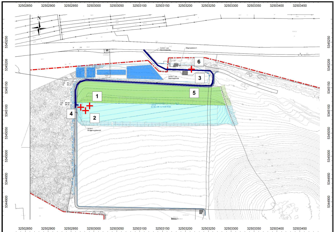
Abb. 5: Lage der Quellen Betriebsabschnitt BA 0.2 – IO1
