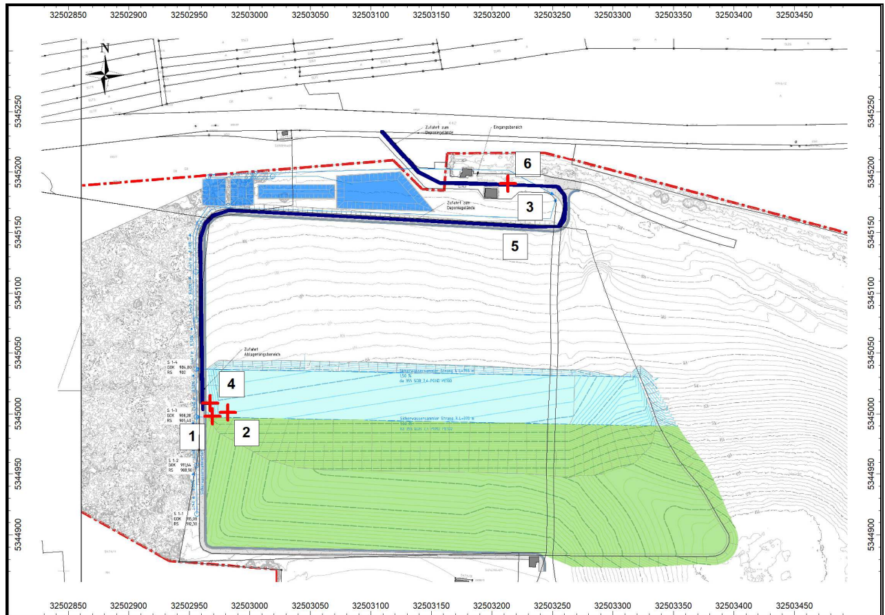
Abb. 19: Lage der Quellen Betriebsabschnitt BA 1.3 – IO3
