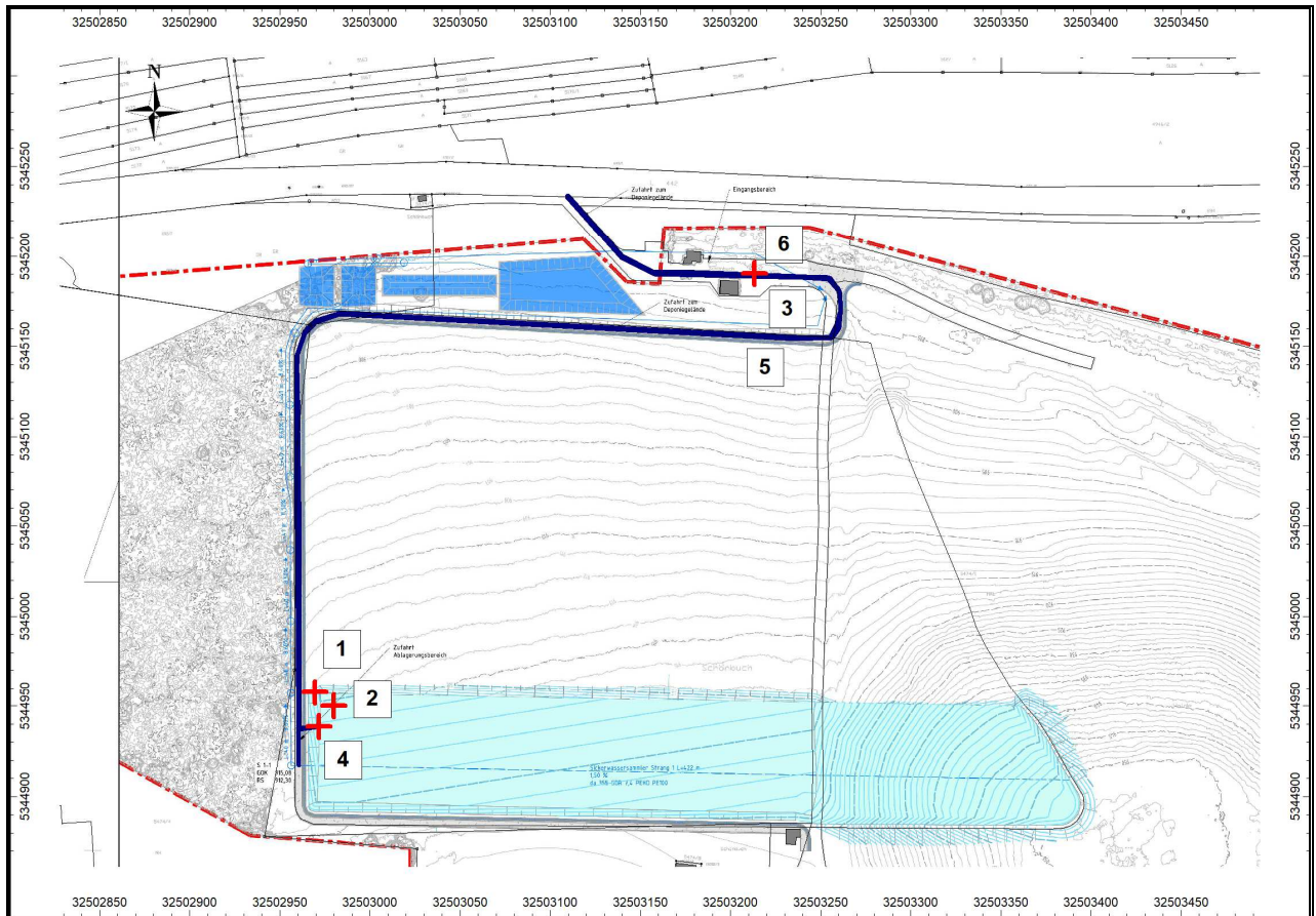
Abb. 12: Lage der Quellen Betriebsabschnitt BA 1.1 – IO2
