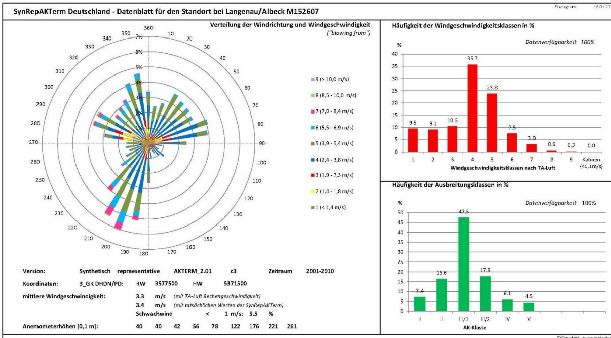
Abbildung 8-1: Verwendete Windverteilung
