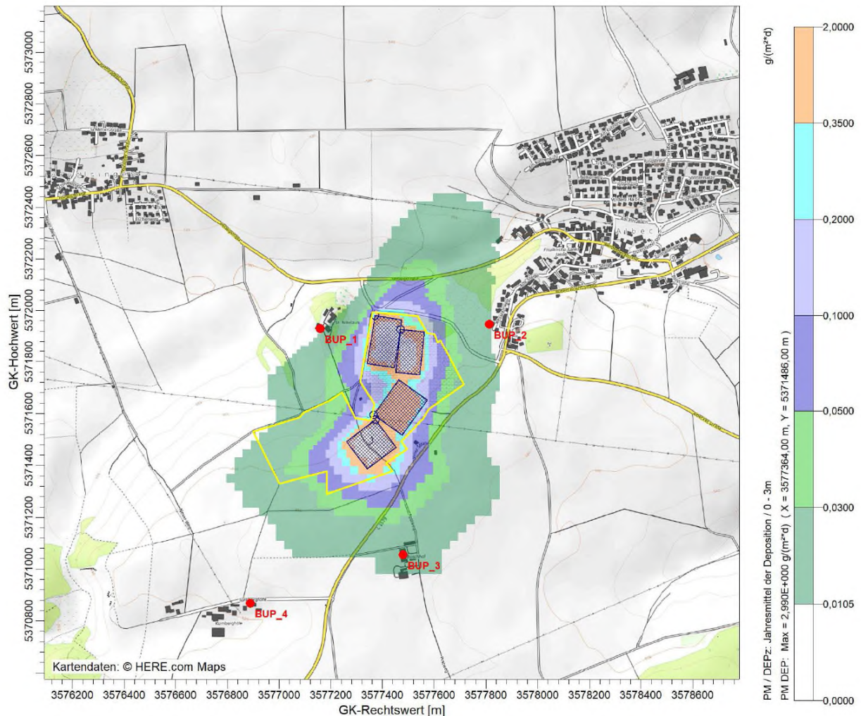
Abbildung 5: Immissionen durch Staubbiederschlag des Betriebs Eckle (Jahresmittel in \text{mg}/\text{m}^2 \text{ d} ) – berechnet als Daueremission
