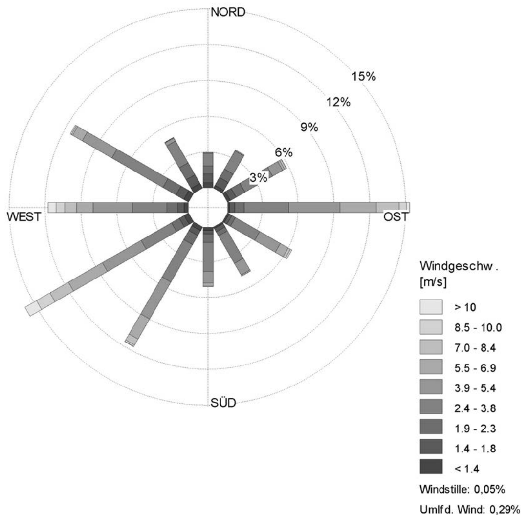
Abbildung 8. Windrichtungshäufigkeitsverteilung der DWD-Station Klippeneck 2015 [8].
