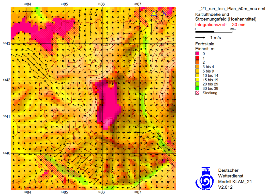
Abbildung 22. Kaltluftströmungsfeld und Kaltluftschichtdicken zu Beginn einer Kaltluftsituation im Umgriff um den Steinbruch im Planfall , umliegende Ortschaften rot schraffiert.
