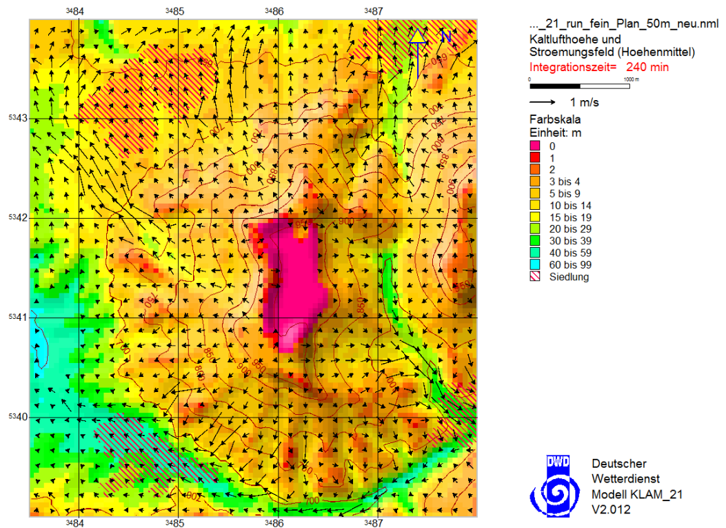
Abbildung 24. Kaltluftströmungsfeld und Kaltluftschichtdicken bei voll ausgebildeter Kaltluft im Umgriff um den Steinbruch im Planfall , umliegenden Ortschaften rot schraffiert.
