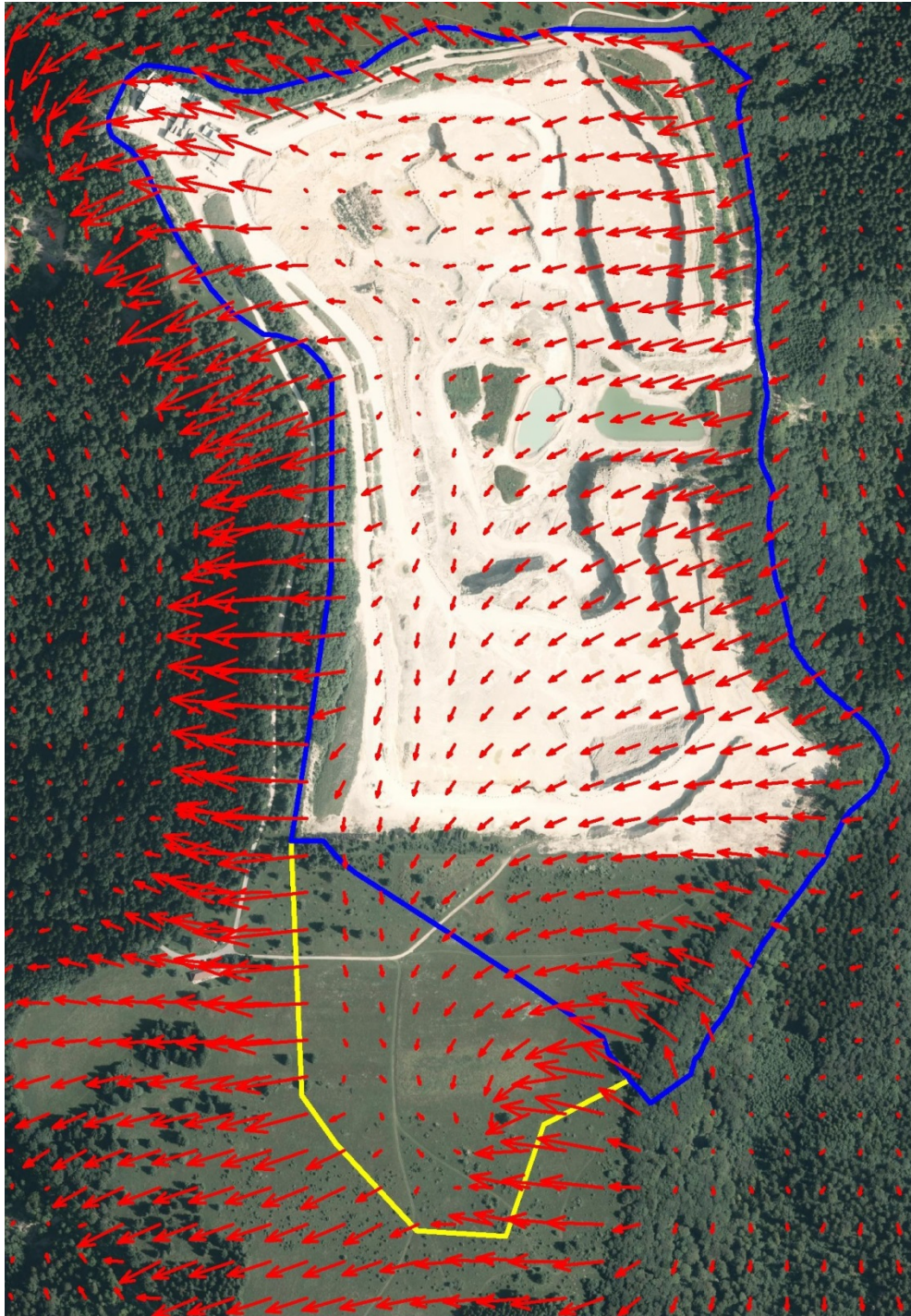
Abbildung 12. Windfeld in 10 m Höhe in der Umgebung des Steinbruchs im Planfall bei einer Anströmung aus 90° (genehmigte Abbaufäche blau umrandet, geplante Erweiterungsfläche gelb umrandet).
