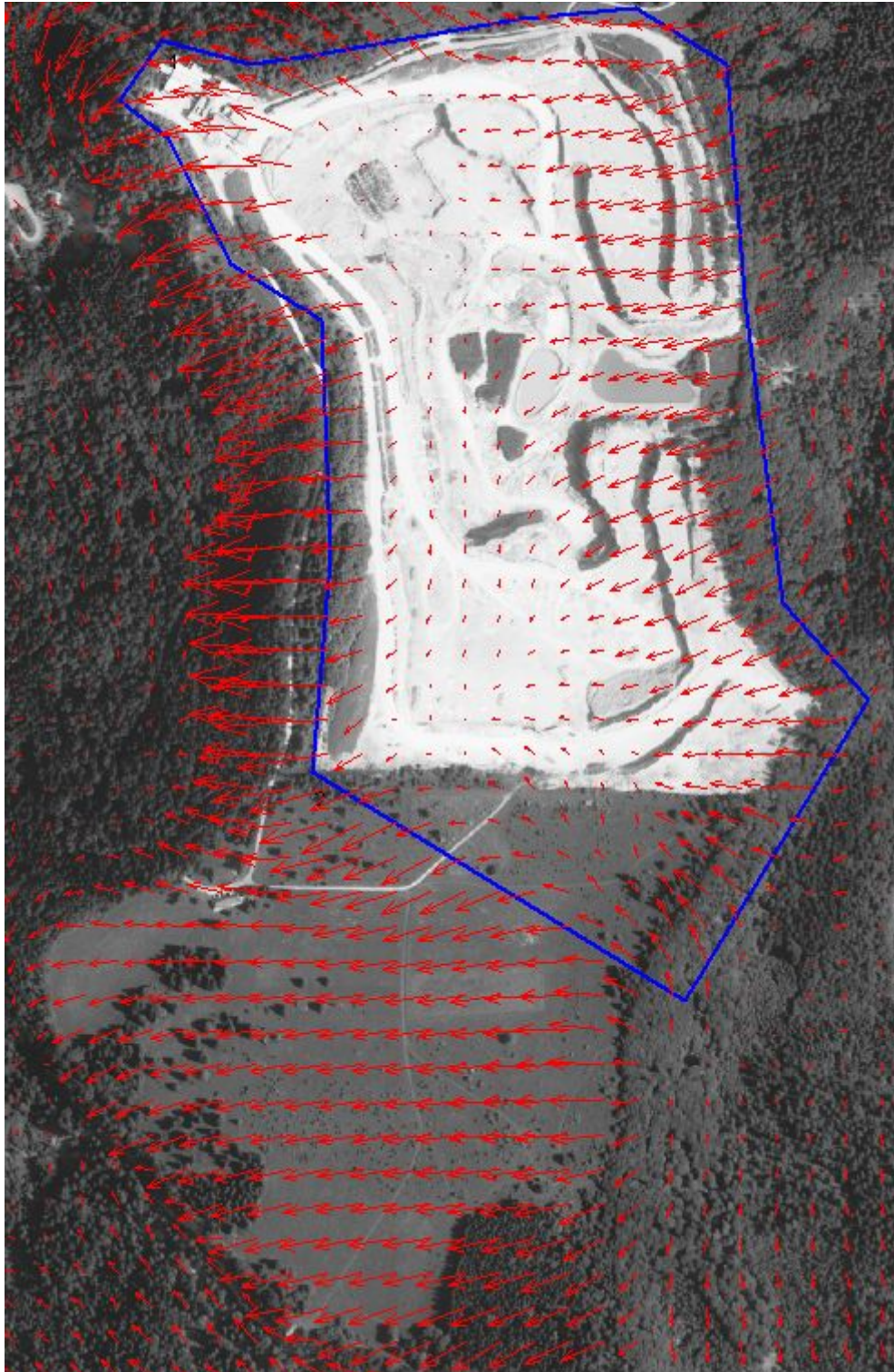
Abbildung 11. Windfeld in 10 m Höhe in der Umgebung des Steinbruchs im genehmigten Zustand bei einer Anströmung aus 90° (genehmigte Abbaufäche unmaßstäblich in blau skizziert).
