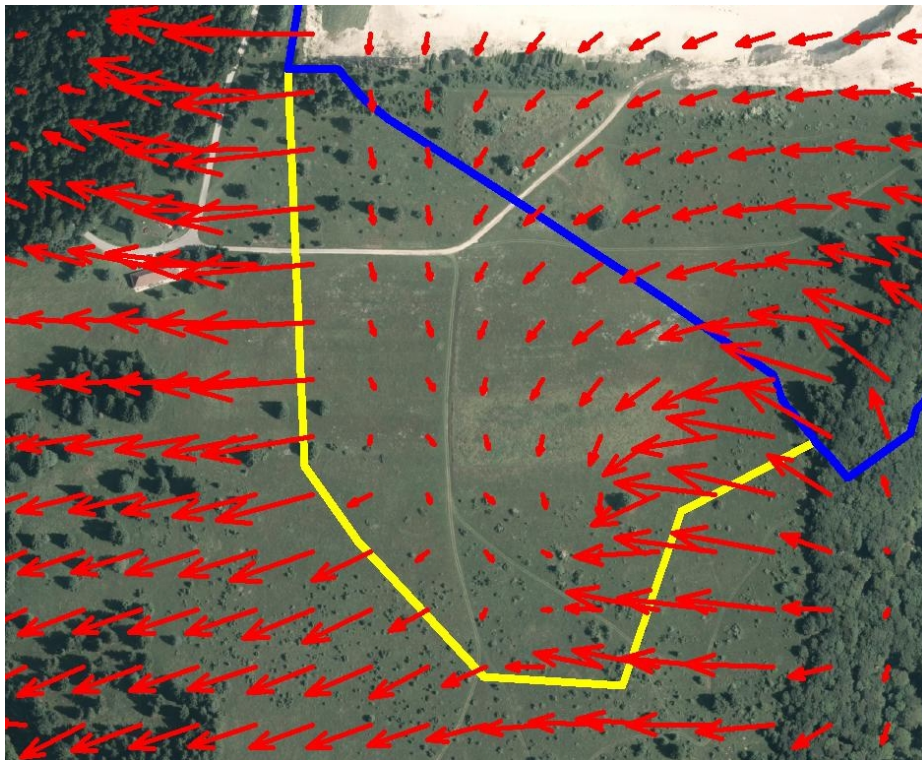
Abbildung 13. Windfeld in 10 m Höhe im Bereich der Süderweiterung des Steinbruchs oben im genehmigten Zustand und unten im Planfall bei einer Anströmung aus 90° (genehmigte Abbaufläche unmaßstäblich in blau skizziert).
