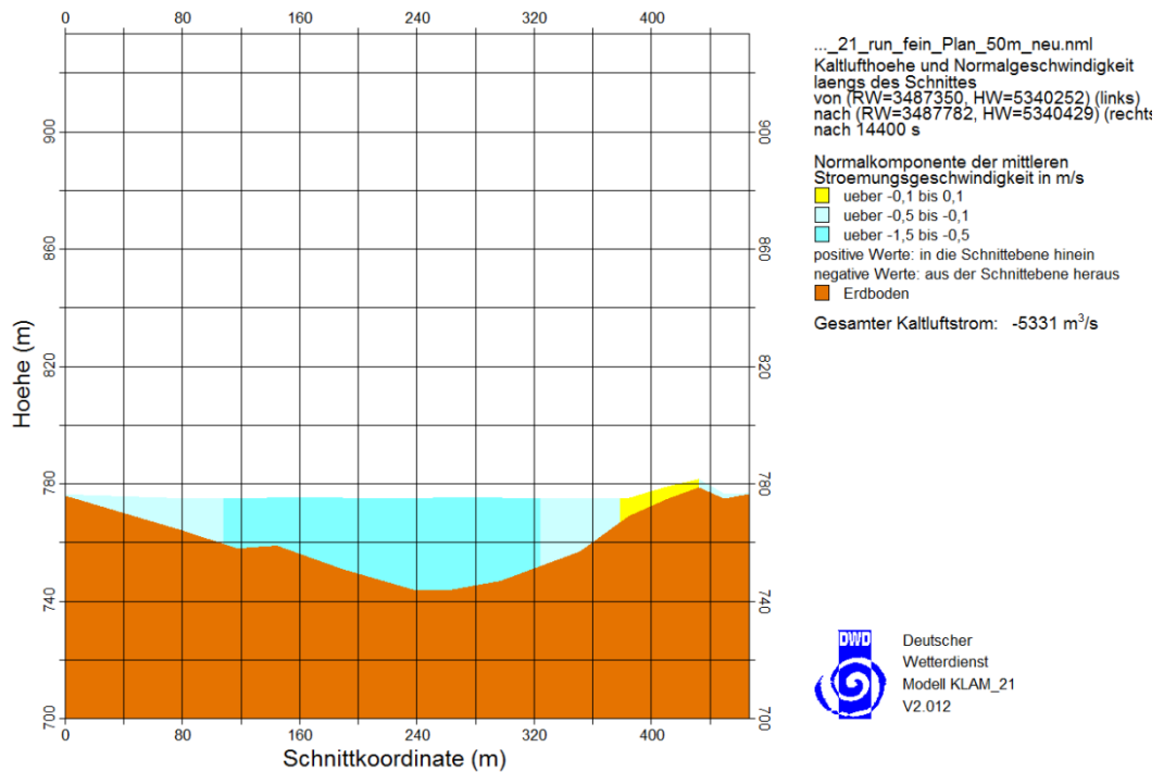
Abbildung 27. Kaltfluthöhe, Fließgeschwindigkeit und bilanzierter Kaltluftstrom entlang von Schnitt 2 (von West nach Ost), oben genehmigter Zustand und unten Planfall.
