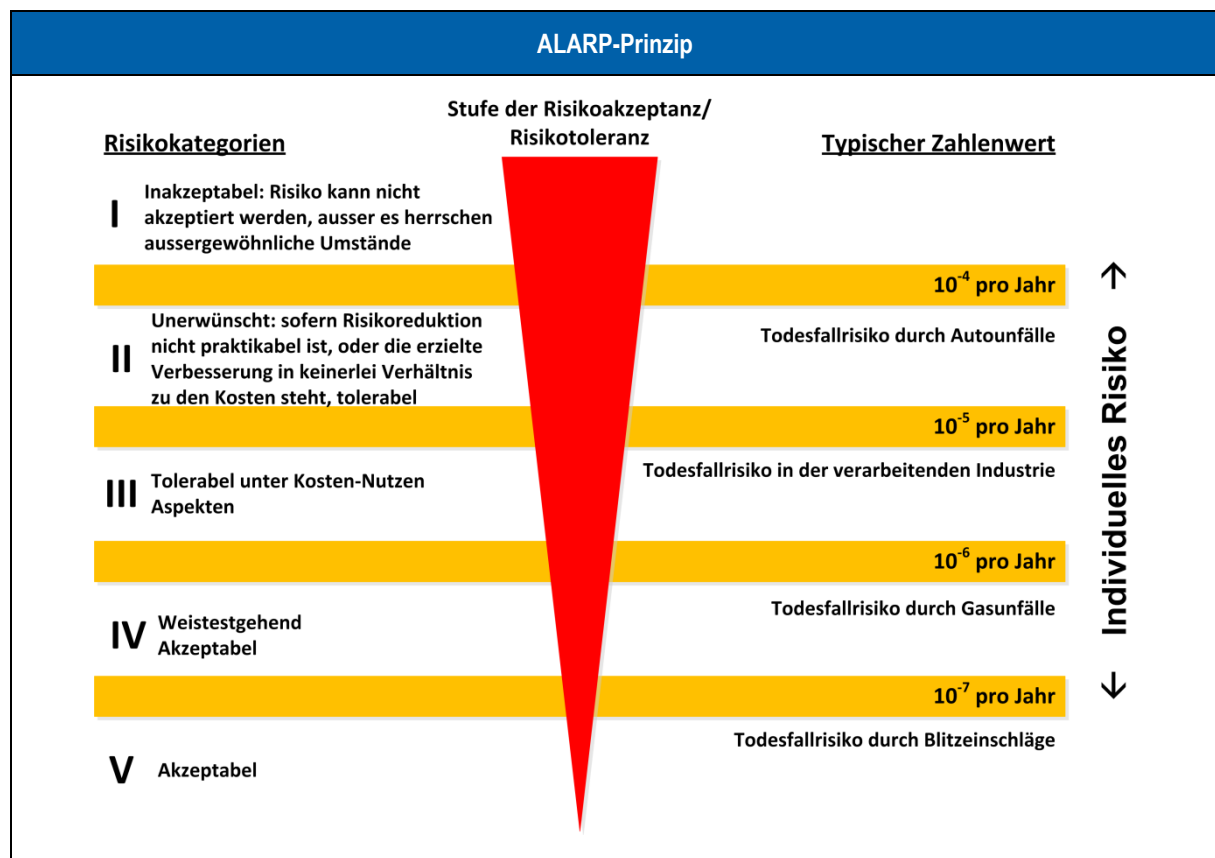
Abbildung 13: ALARP-Prinzip
