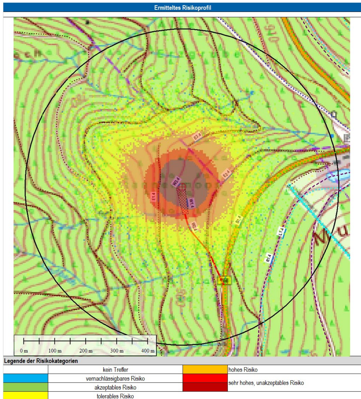
Abbildung 9: Übersicht zur Lage der Untersuchungsobjekte an der WEA_LAU inklusive des Umkreises von 505.5 m um die WEA herum und des Risikoprofils für das kollektive Risiko für Autofahrer auf der B500.
