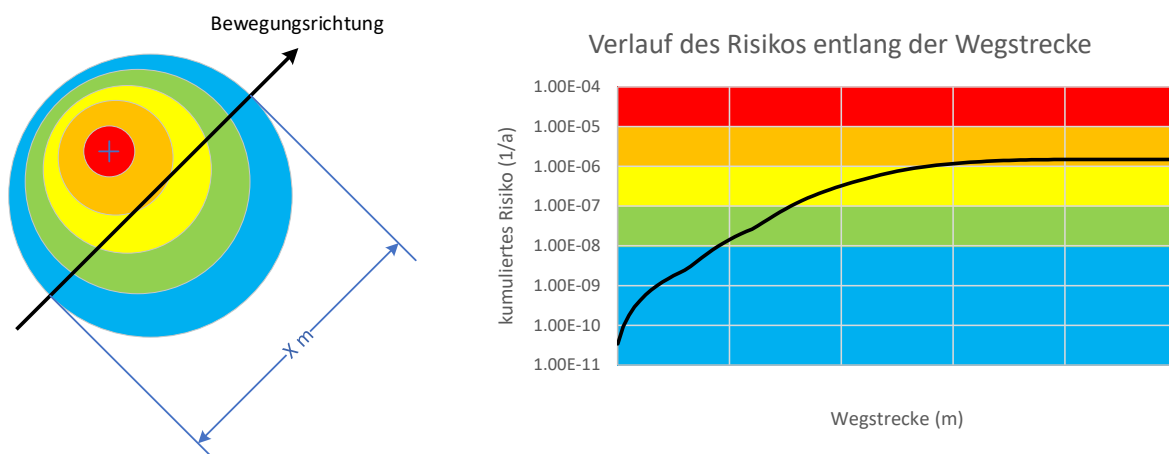
Abbildung 5: Schematische Darstellung, wie sich das Risiko für einen Fußgänger entlang einer Wegstrecke entwickelt. Durchschreitet der Fußgänger den gesamten Gefährdungsbereich von X Meter so hat er sich in dem oben links eingezeichneten Weg (schwarzer Pfeil) in Summe einem hohen Risiko ausgesetzt. Wird der Weg verlegt, sodass er den orange schraffierten Bereich nicht mehr berührt, sinkt das aufsummierte Risiko in den tolerablen Bereich ab.
