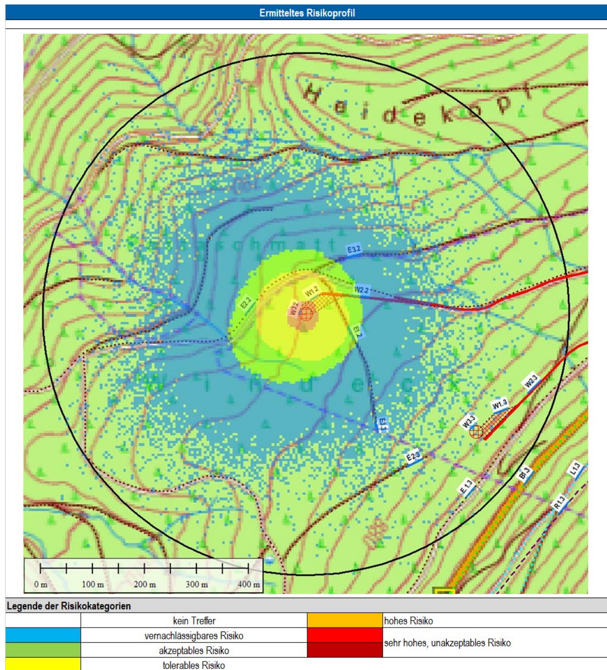
Abbildung 7: Übersicht zur Lage der Untersuchungsobjekte an der WEA2_OTT inklusive des Umkreises von 505.5 m um die WEA herum und des Risikoprofils für das individuelle Risiko für Fußgänger auf gelegentlich benutzten Wegen.
