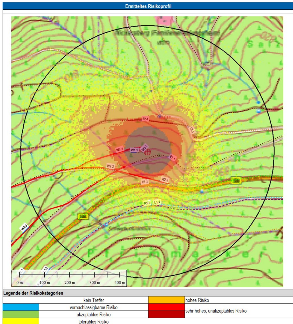
Abbildung 6: Übersicht zur Lage der Untersuchungsobjekte an der WEA1_OTT inklusive des Umkreises von 505.5 m um die WEA herum und des Risikoprofils für das kollektive Risiko für Autofahrer auf der B500.
