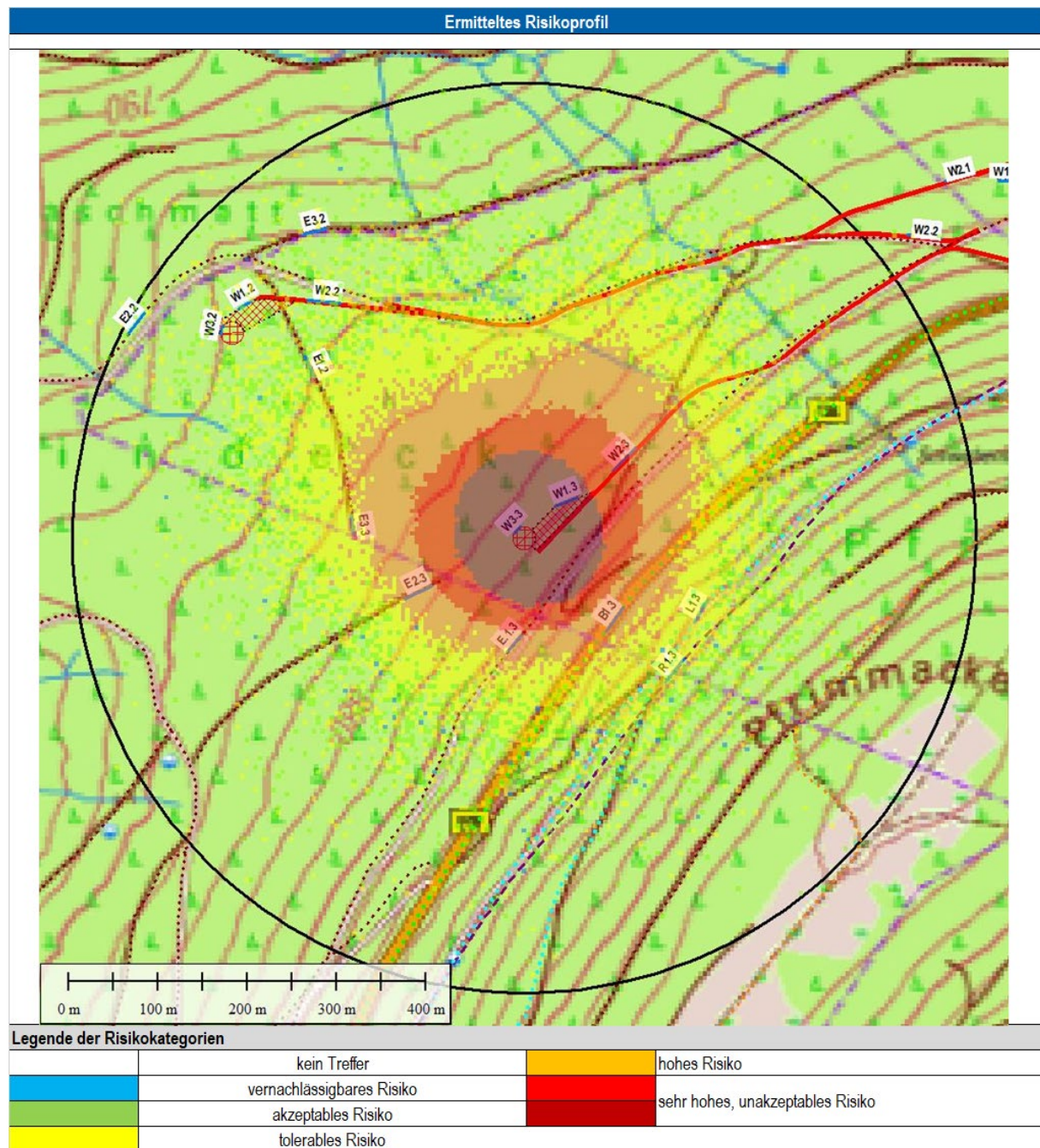
Abbildung 8: Übersicht zur Lage der Untersuchungsobjekte an der WEA3_OTT inklusive des Umkreises von 505.5 m um die WEA herum und des Risikoprofils für das kollektive Risiko für Autofahrer auf der B500.
