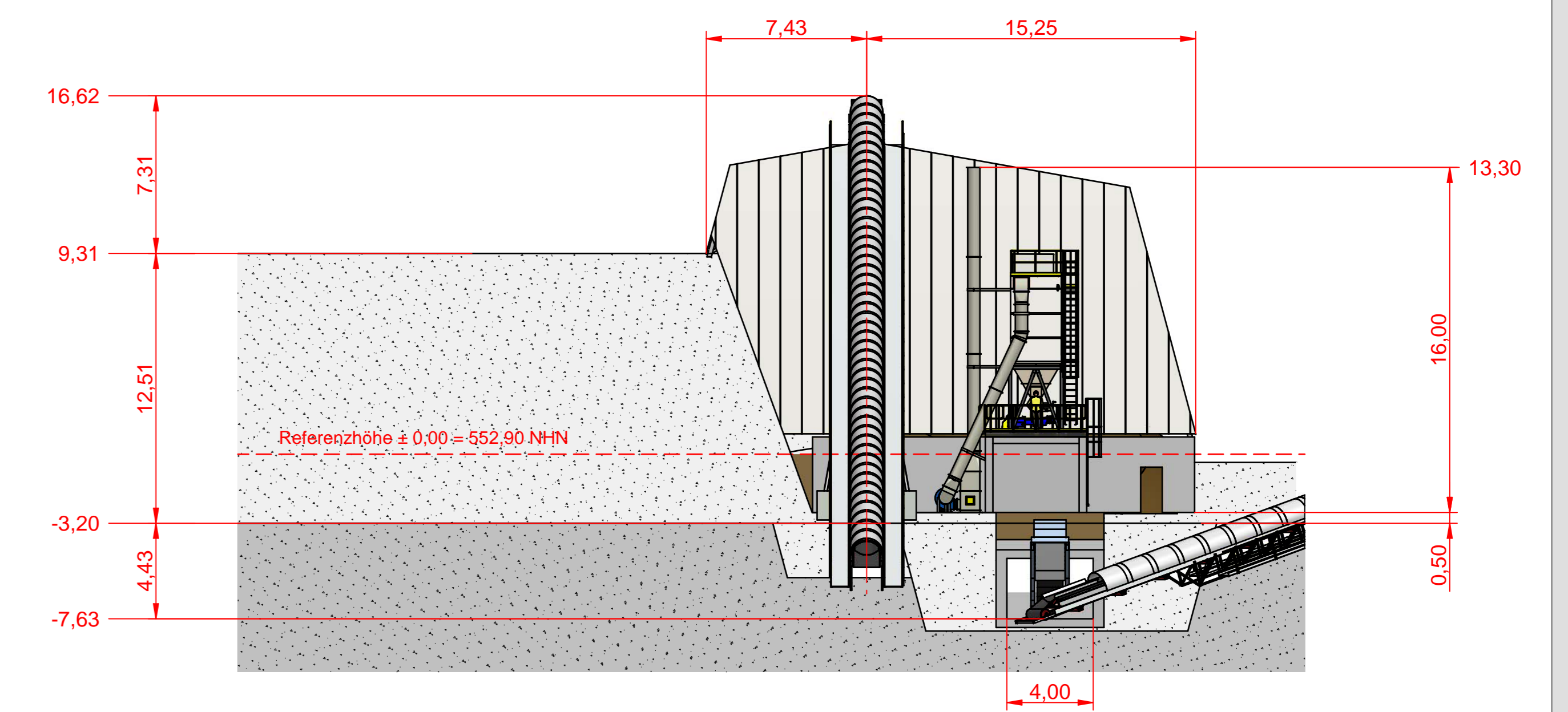
Ansicht West
