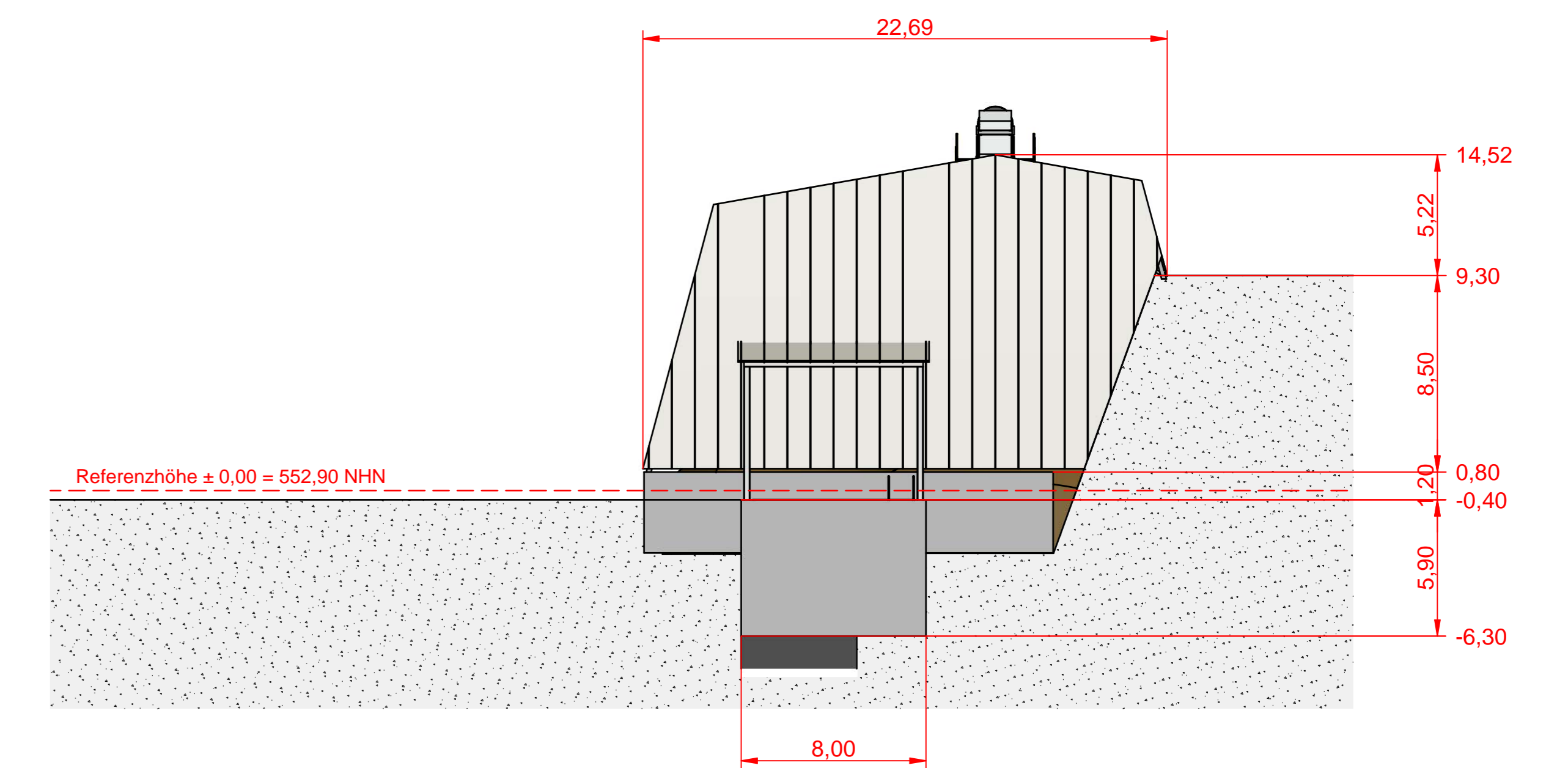
Ansicht Ost
