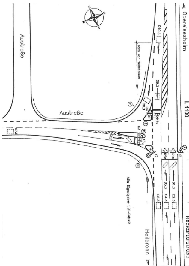
Abbildung 14: Lageplan LSA L1100/ Austraße
