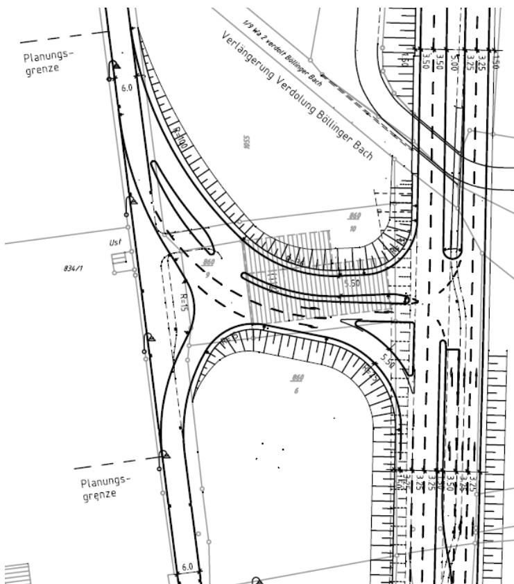
Abbildung 18: Lageplan LSA L1100/ Wimpfener Straße (Höhe Tierheim) – Planfall 2
